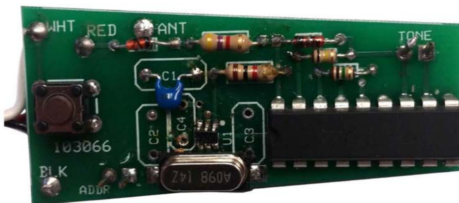
Top Side
