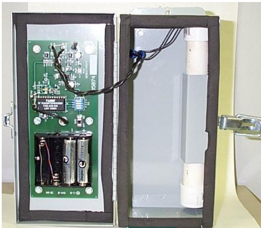
EUT open
