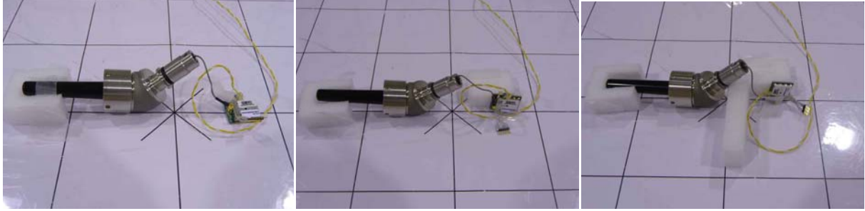
(module: X-axis, antenna: Z-axis) (module: Y-axis, antenna: Z-axis) (module: Z-axis, antenna: Z-axis)
