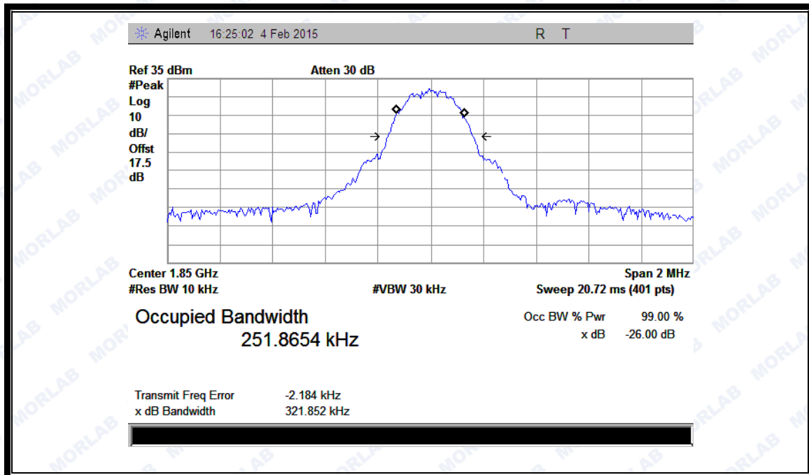
(Plot J: GPRS 1900MHz Channel = 512)
