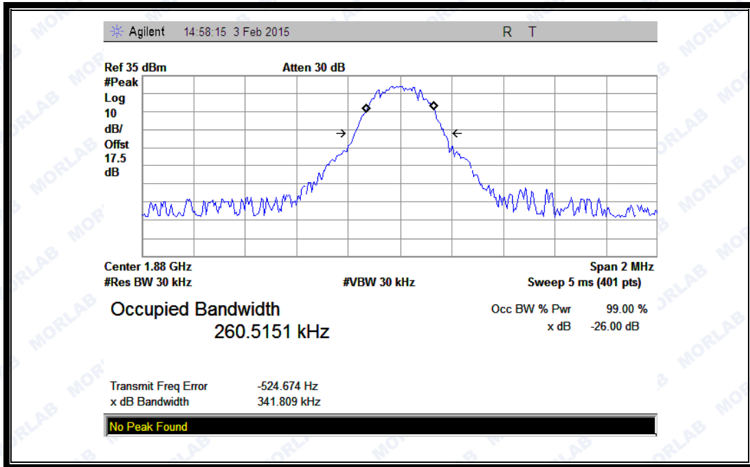
(Plot E: GSM 1900MHz Channel = 661)
