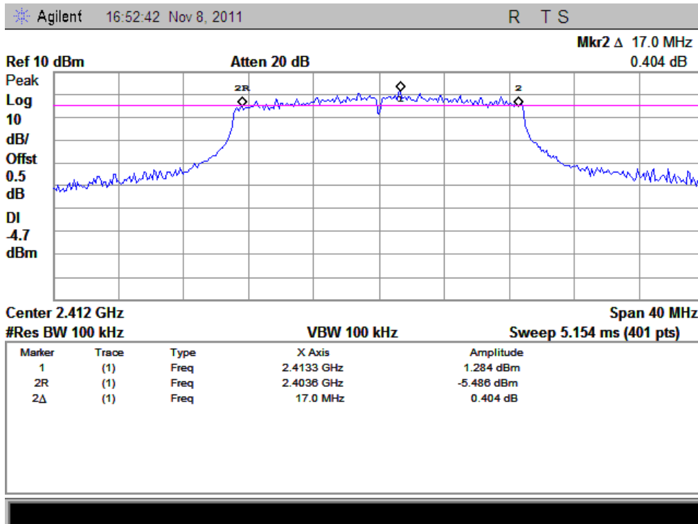
(Plot A: Chain1_Channel 1: 2412MHz)
