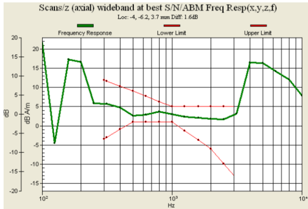
Fig. 9.1 GSM850 Ch128
