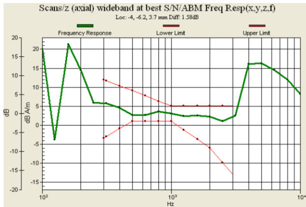
Fig. 9.3 GSM850 Ch251
