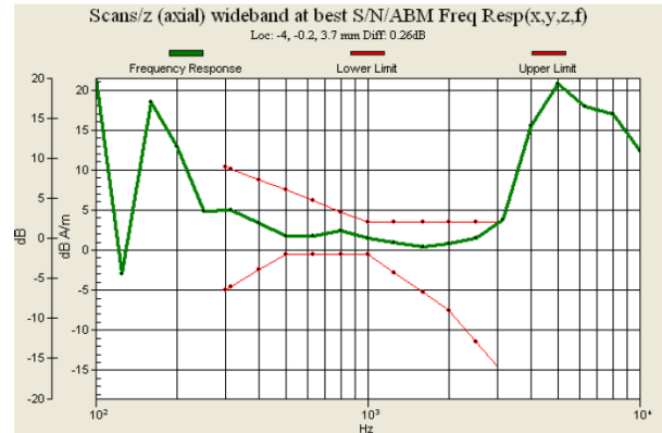
Fig. 9.8 WCDMA Band IV Ch1413
