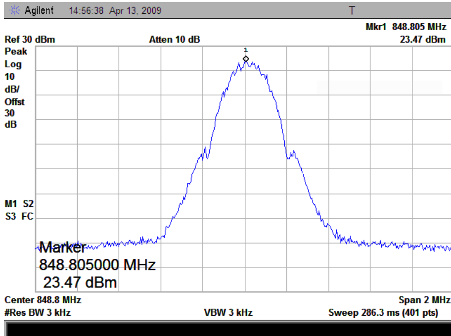
(Plot B: GSM 850MHz Channel = 251)
