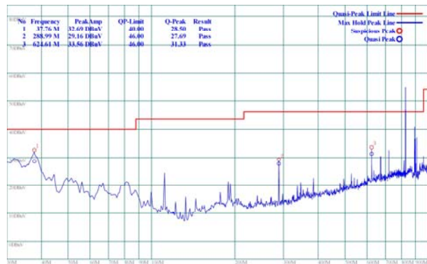
(Plot A: Test Antenna Vertical)
