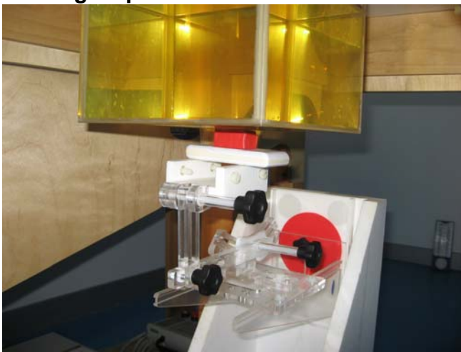
Fig.7 spacer 1.5cm
