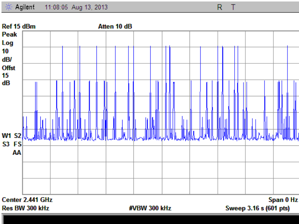
(Plot E: DH3 @ \pi/4 -DQPSK)
