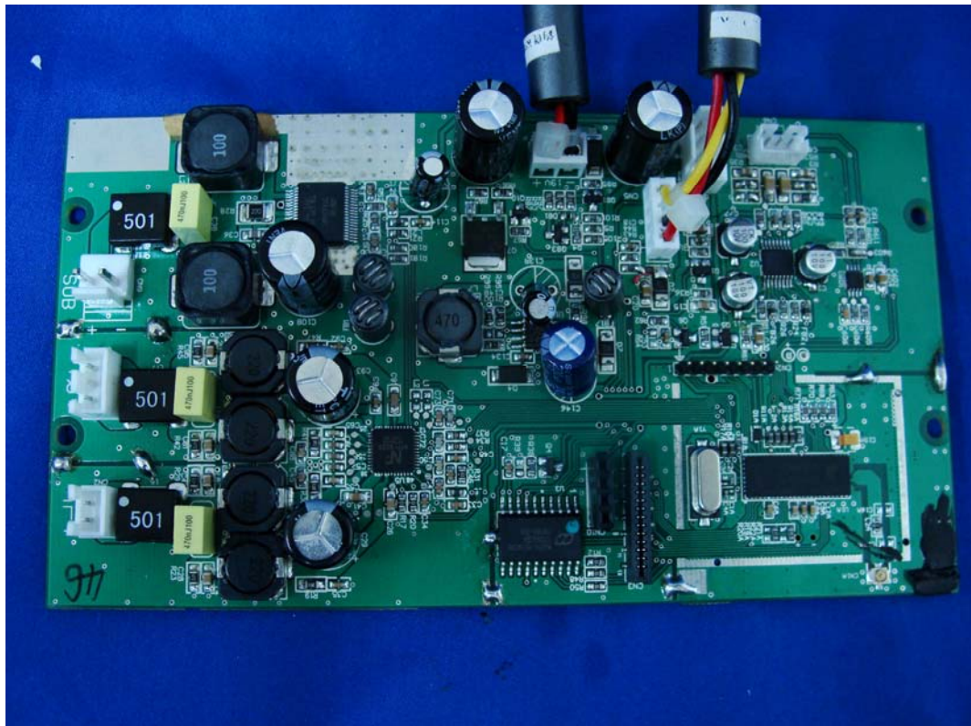
(16) EUT Photo (RF Chip)
