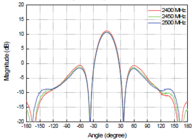
V-plane Co-polar. Pattern
