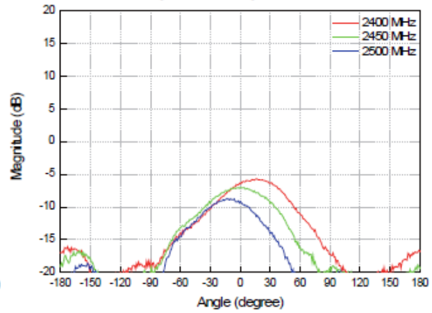
H-plane Cross-polar. Pattern
