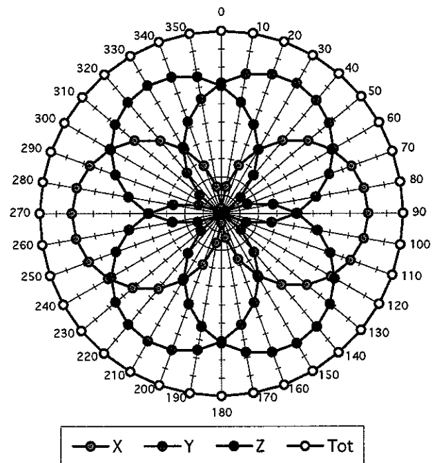
f = 900 MHz, TEM cell if110
