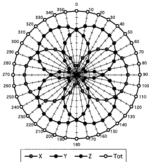
f = 300 MHz, TEM cell if110
