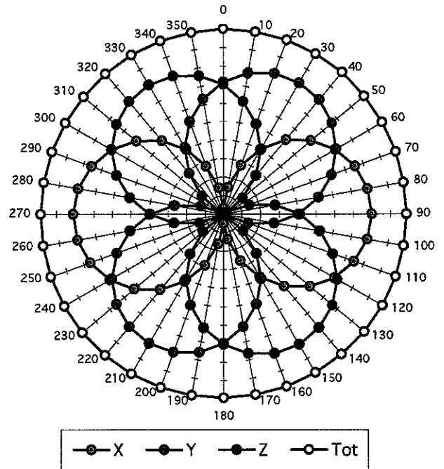
f = 100 MHz, TEM cell if110
