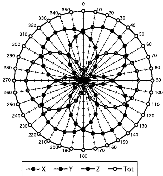
f = 30 MHz, TEM cell if110
