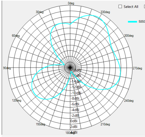
5850MHZ V-pol
