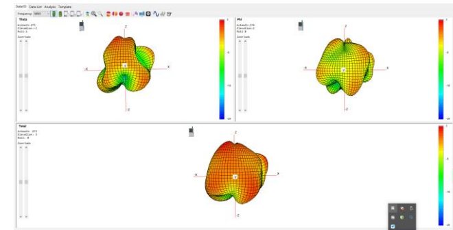
5850MHZ 3D
