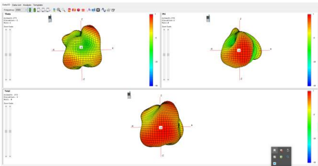
2500MHZ 3D
