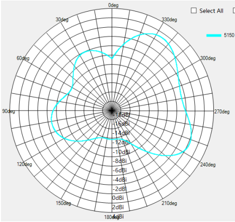
5150MHZ V-pol
