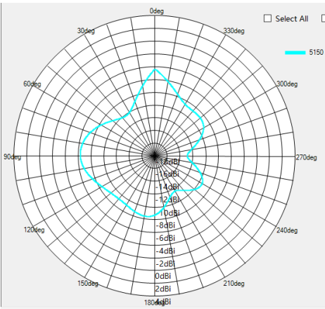
5150MHZ H-pol
