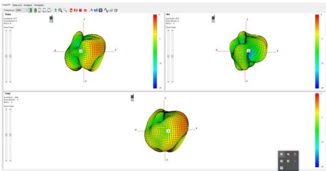
2450MHZ 3D
