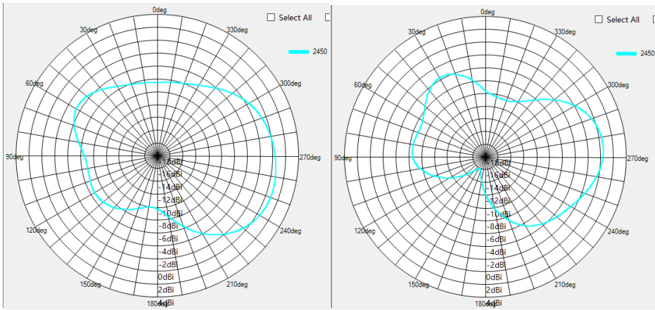
2450MHZ V-pol
