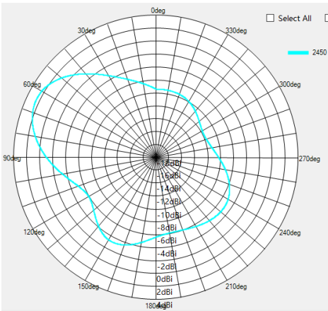
2450MHZ V-pol
