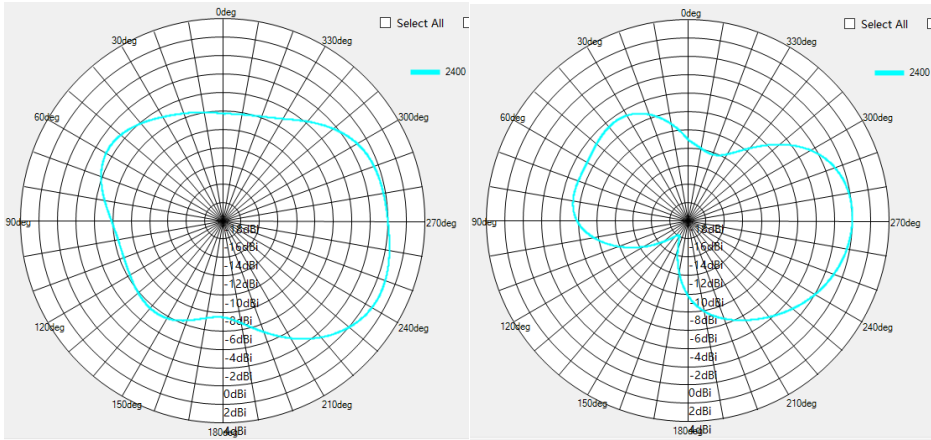
2400MHZ V-pol
