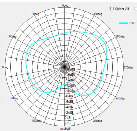
2500MHZ H-pol
