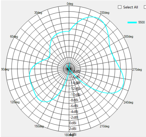
5500MHZ V-pol
