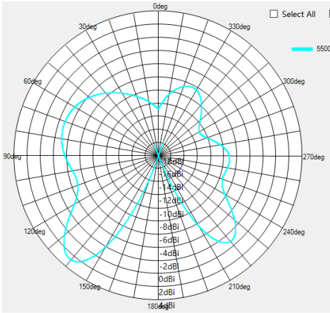
5500MHZ V-pol
