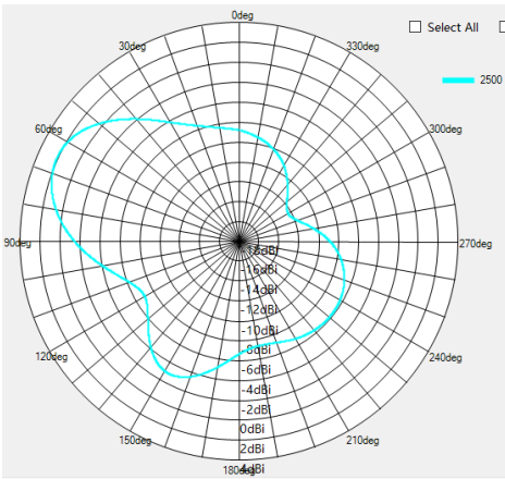
2500MHZ V-pol
