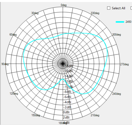
2450MHZ H-pol
