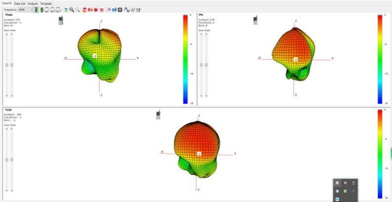
2400MHZ 3D
