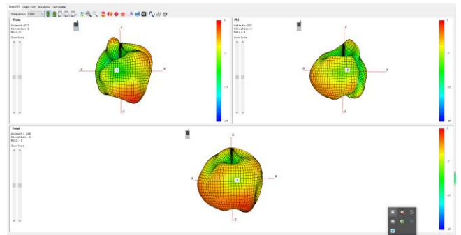
5500MHZ 3D
