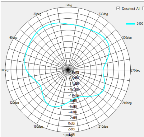
2400MHZ H-pol
