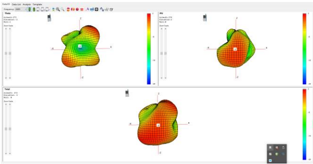
2400MHZ 3D
