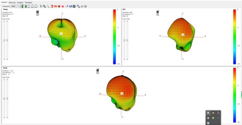
2450MHZ 3D
