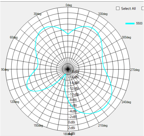
5500MHZ H-pol
