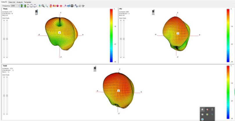
2500MHZ 3D
