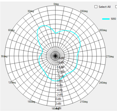
5850MHZ H-pol
