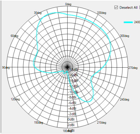
2400MHZ V-pol
