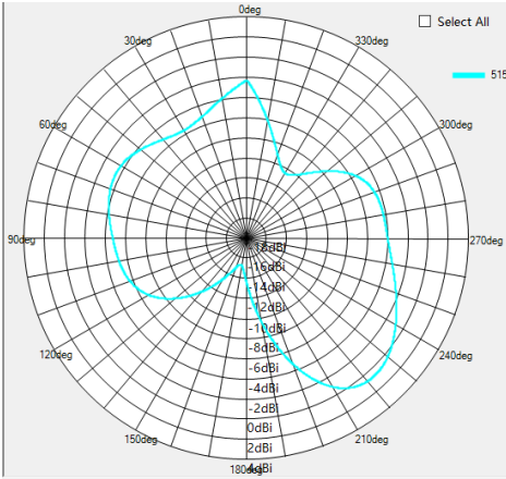
5150MHZ V-pol
