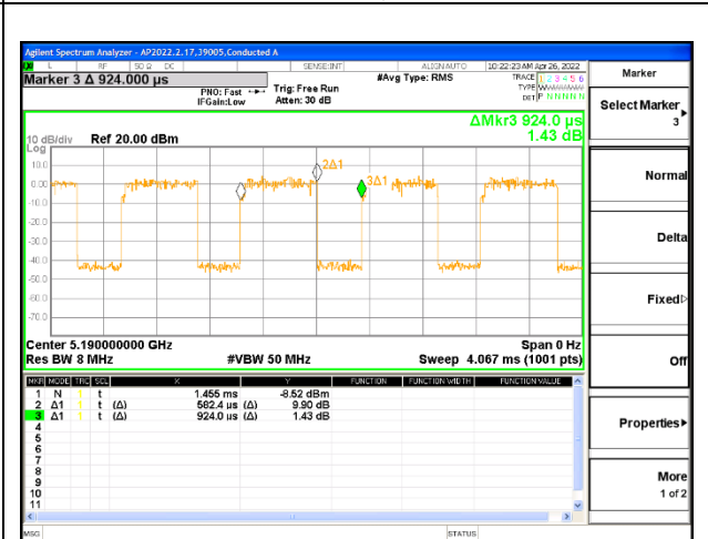
802.11ax HE40 OFDMA, RU size 26T MODE
