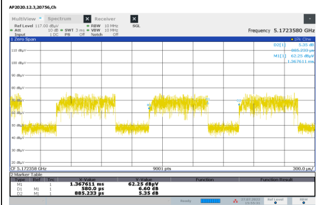
802.11ax HE40 OFDMA, RU size 26T MODE
