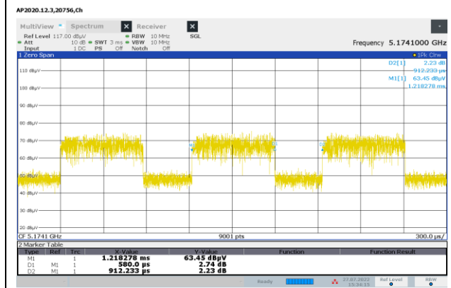
802.11ax HE20 OFDMA, RU size 26T MODE
