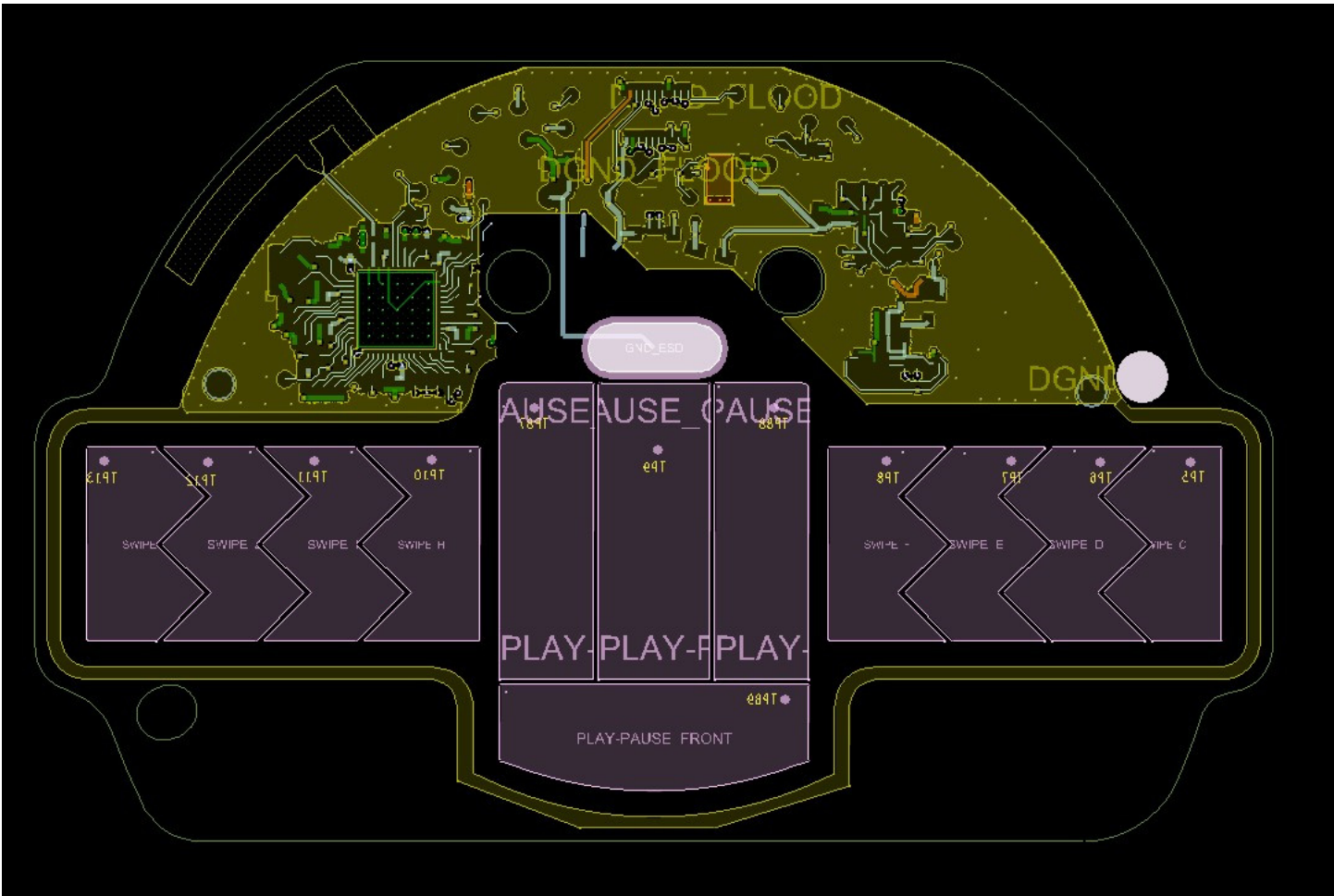
BLE Radio and Antenna
