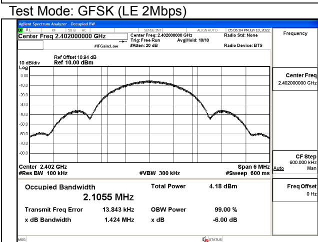
Test Mode:GFSK (LE 2Mbps) MHz
