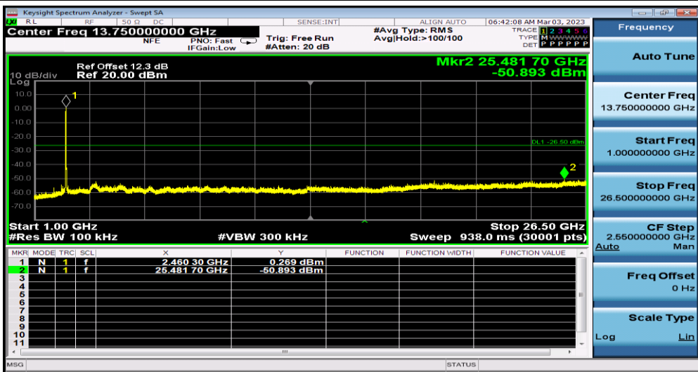
11G_Ant1_2462_1000~26500
