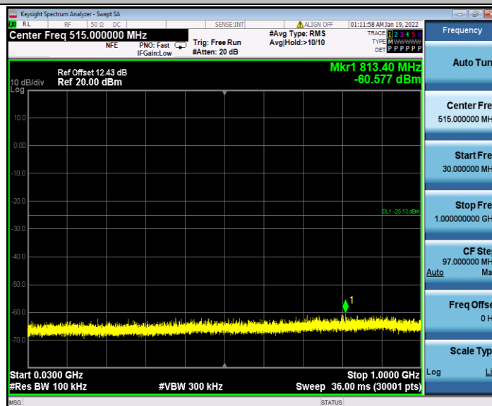
11AX20MIMO_Ant2_2412_30~1000
