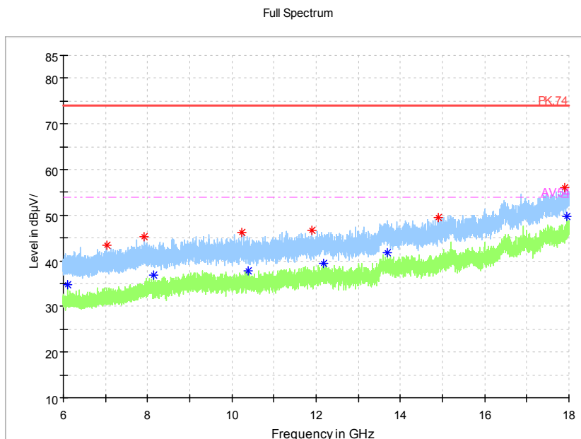
Frequency Range: 6GHz -18GHz Detector: Av mode and PK mode Modulation type: 802.11n(HT40 MIMO)
