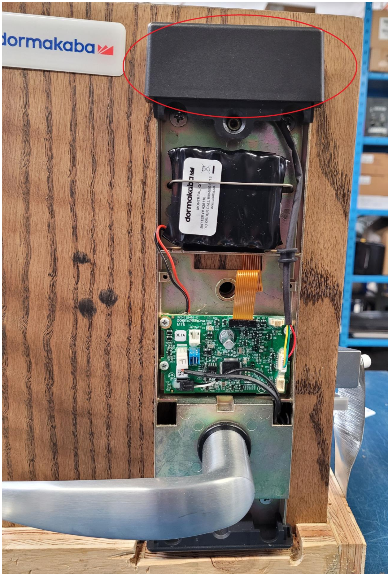
ZigBee module
