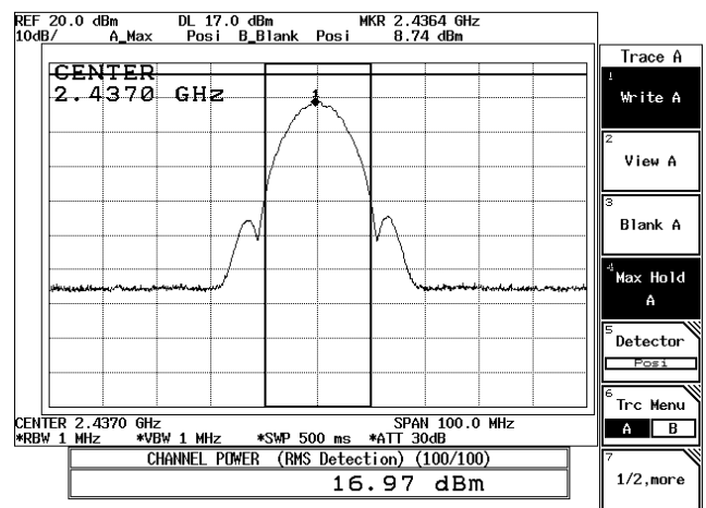
11Mbps-CH 06
