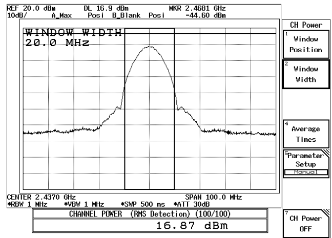
11Mbps-CH 06
