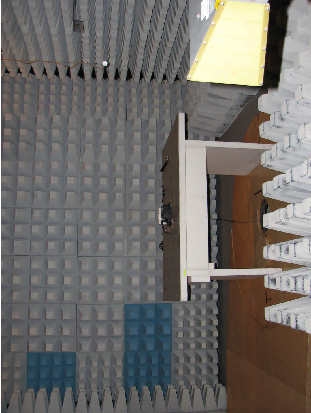
71209emi6.JPG IVTM ECU, testsetup anechoic chamber
