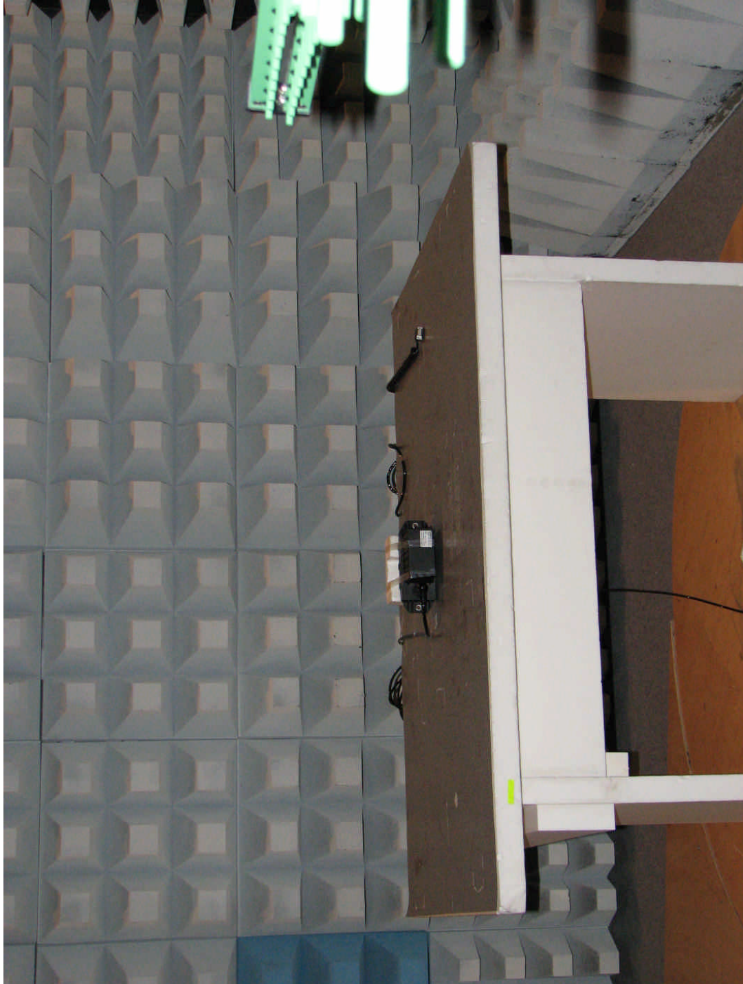
71209emi1.JPG IVTM ECU, testsetup anechoic chamber
