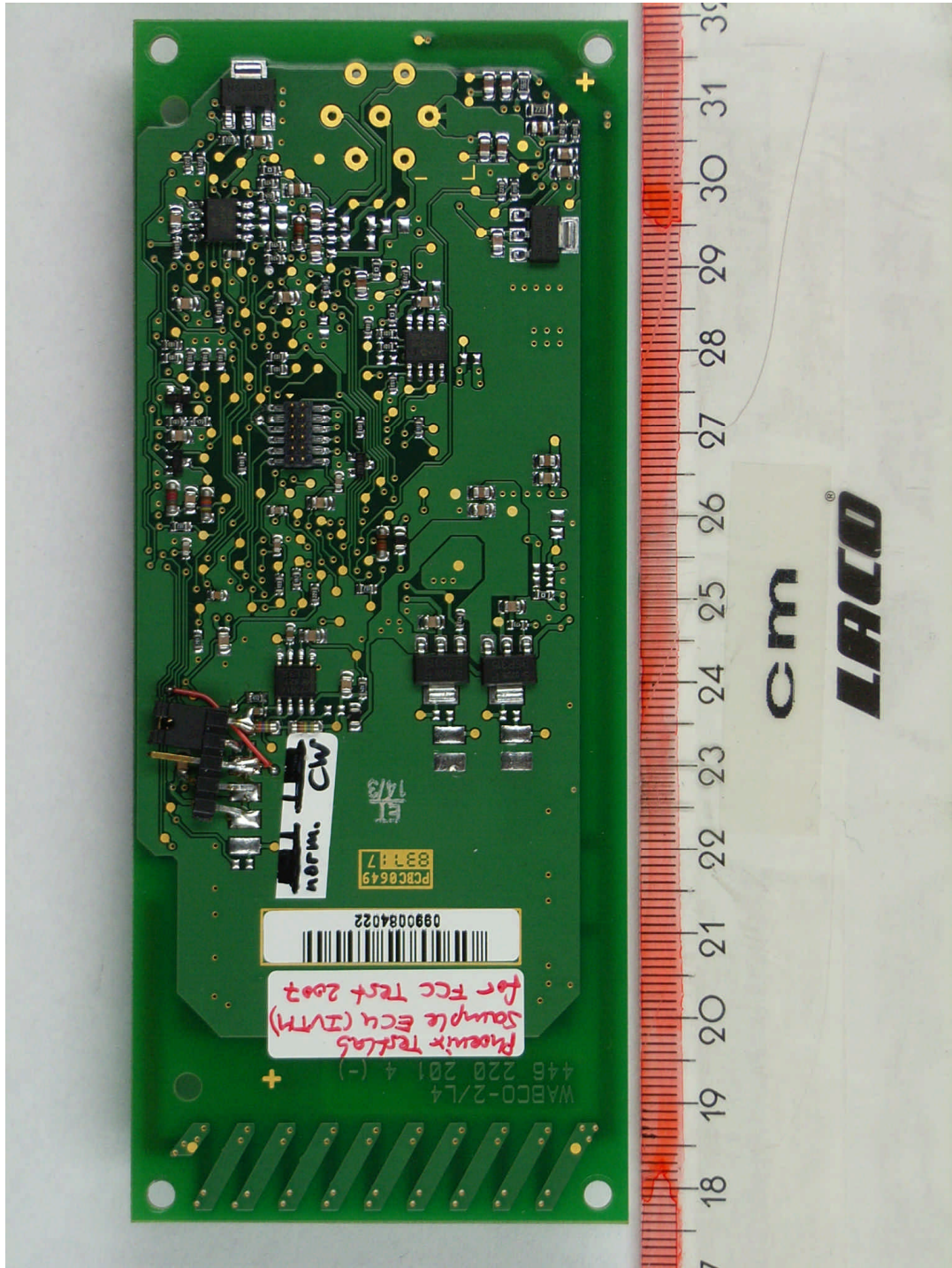
71209eut7.JPG IVTM ECU, pcb bottom view
