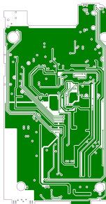
VCC Layer
