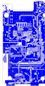
Bottom Layer
