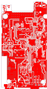
Top Layer
