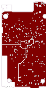
GND Layer
