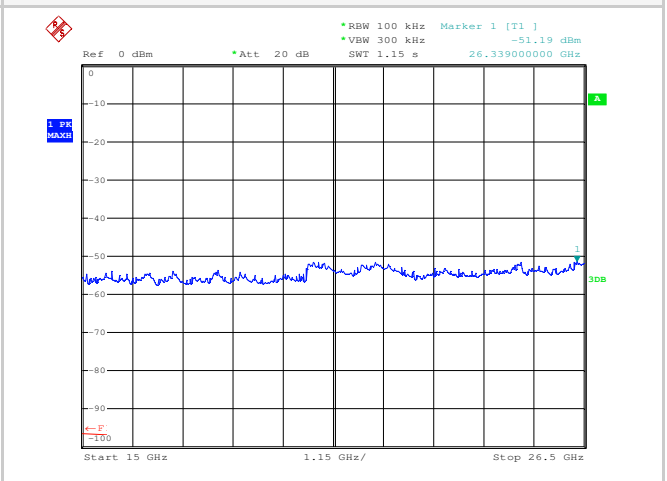
Plot 6 (15÷26.5GHz)
