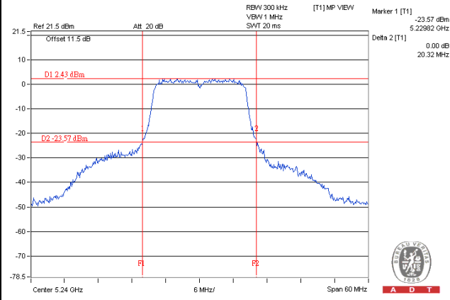
802.11a_CH48
