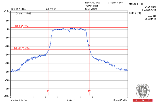
802.11n (HT20)_CH48
