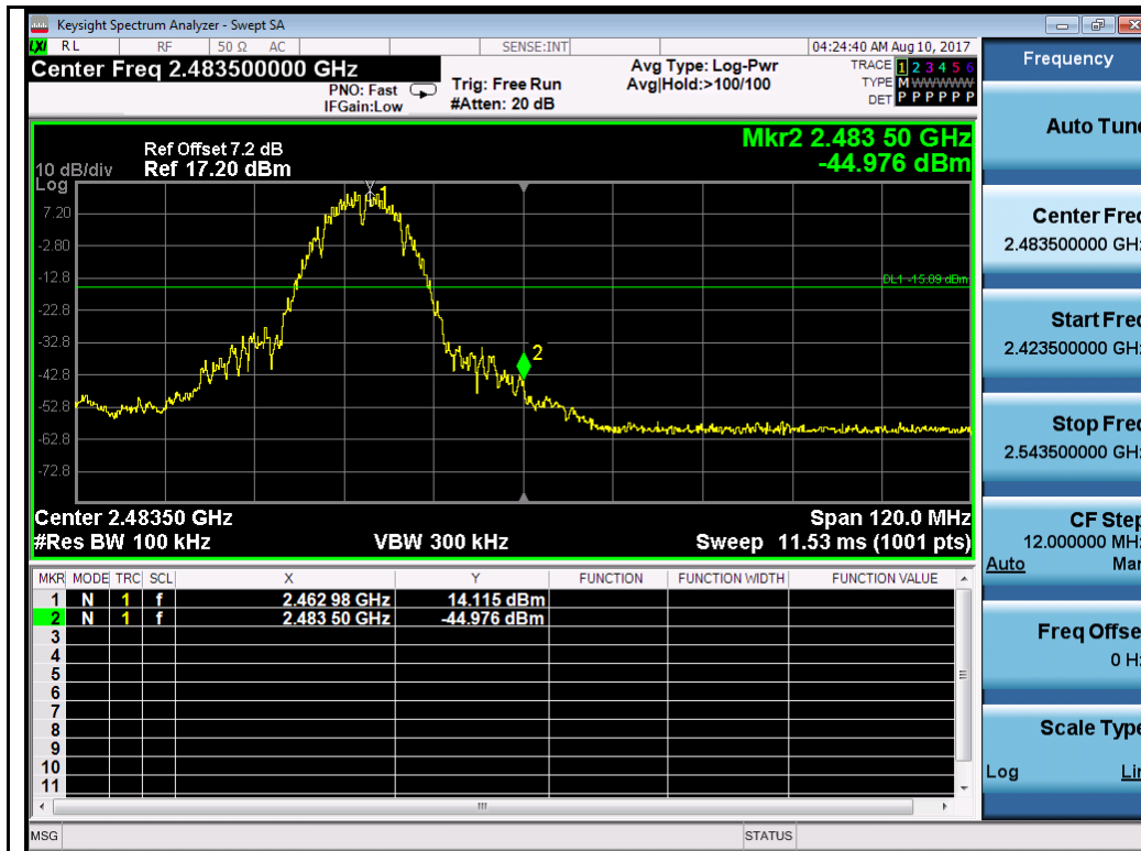
802.11b-2462MHz Chain 2
