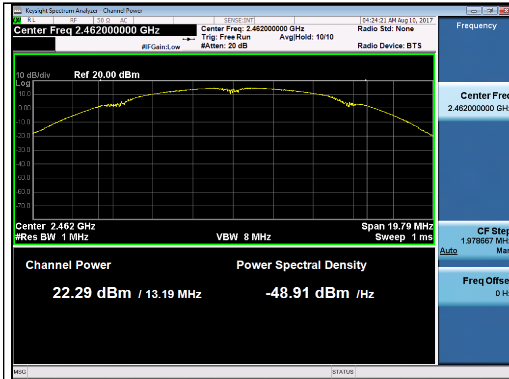
802.11b-2462MHz Chain 2
