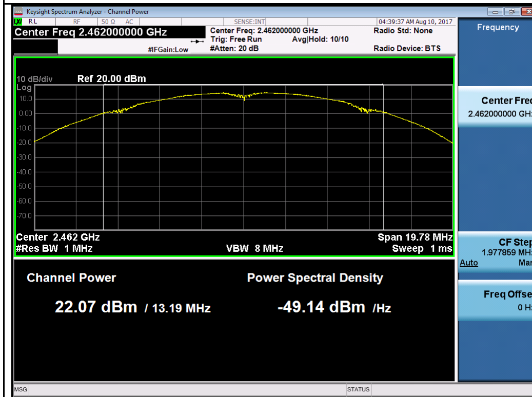
802.11b-2462MHz Chain 3
