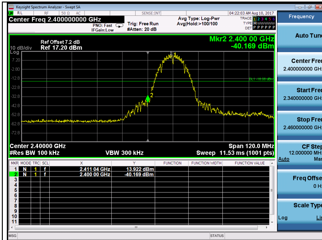
802.11b-2412MHz Chain 2
