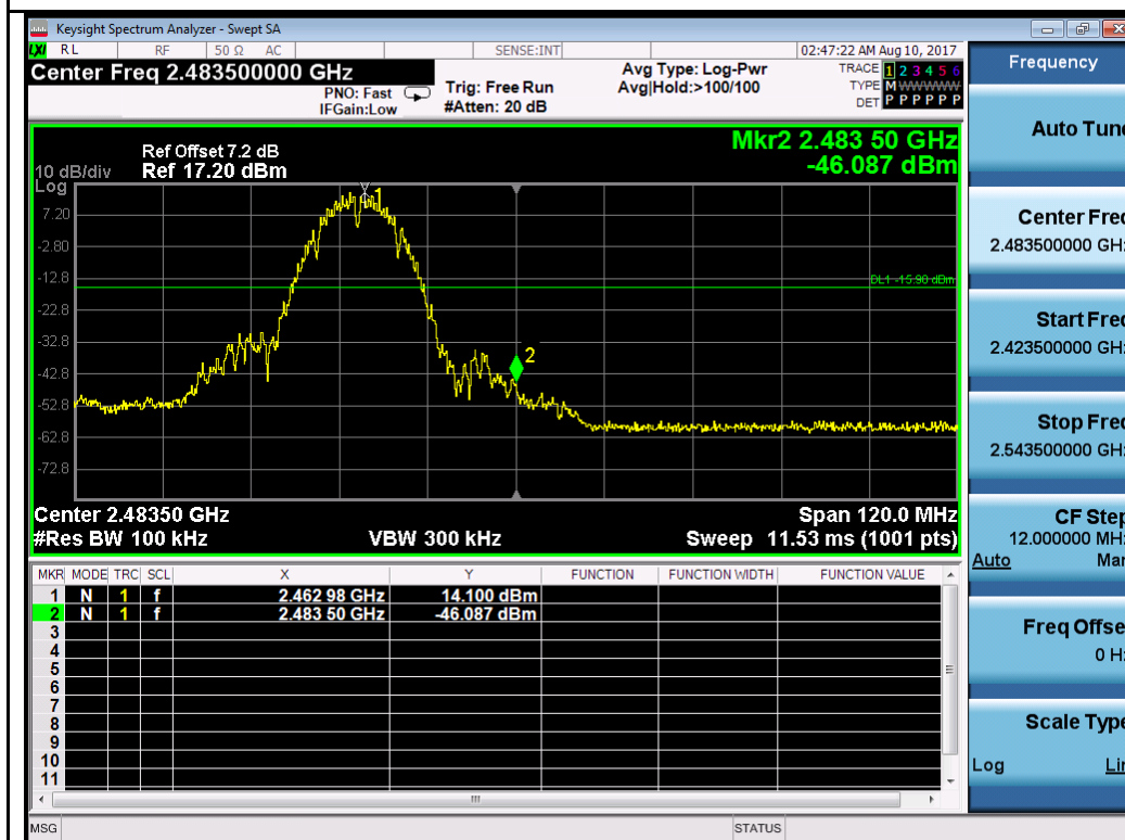
802.11b-2462MHz Chain 1
