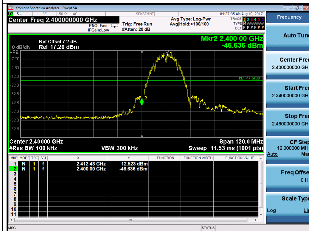
802.11b-2412MHz Chain 3
