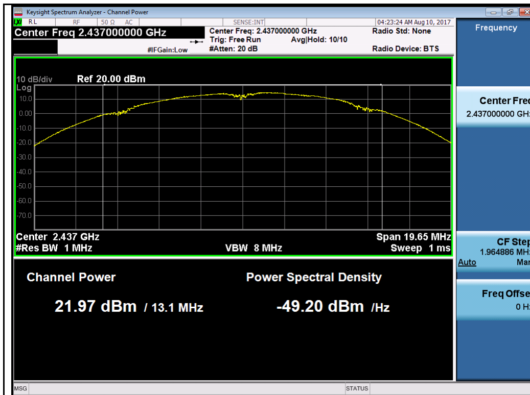
802.11b-2437MHz Chain 2
