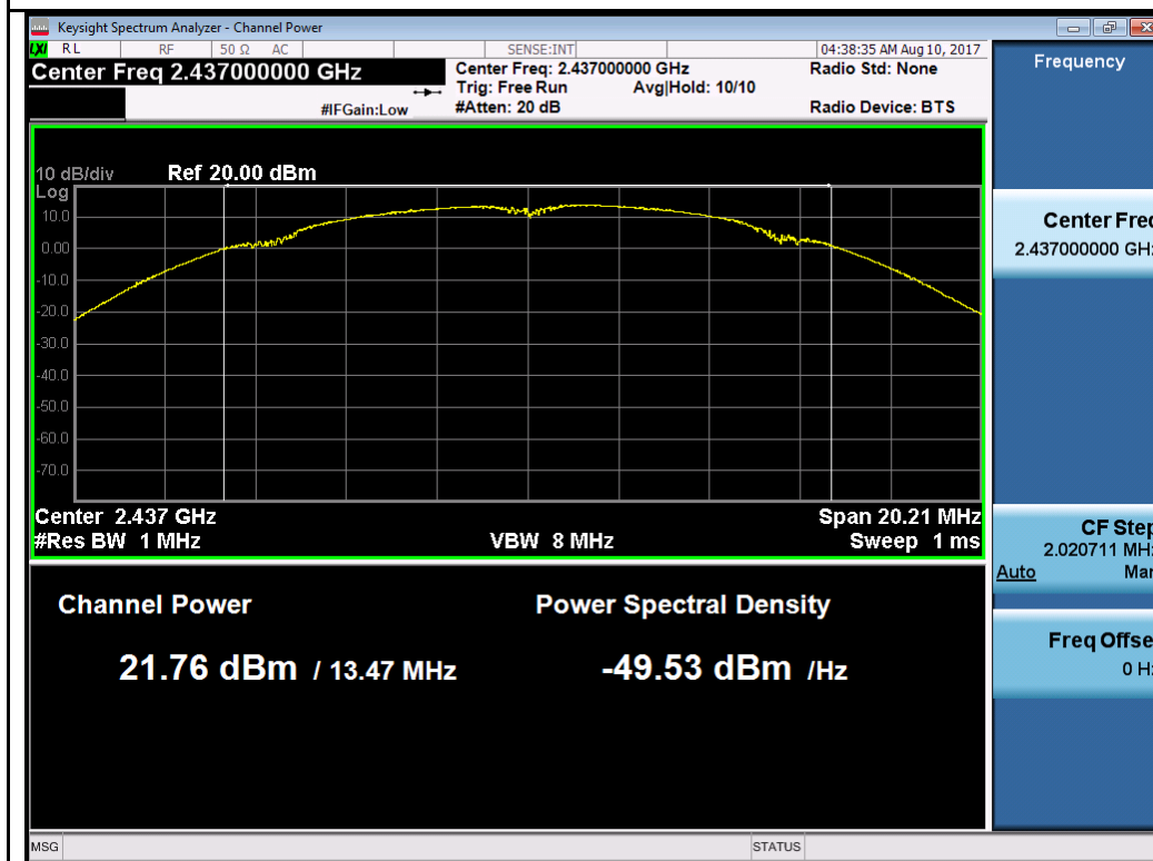
802.11b-2437MHz Chain 3
