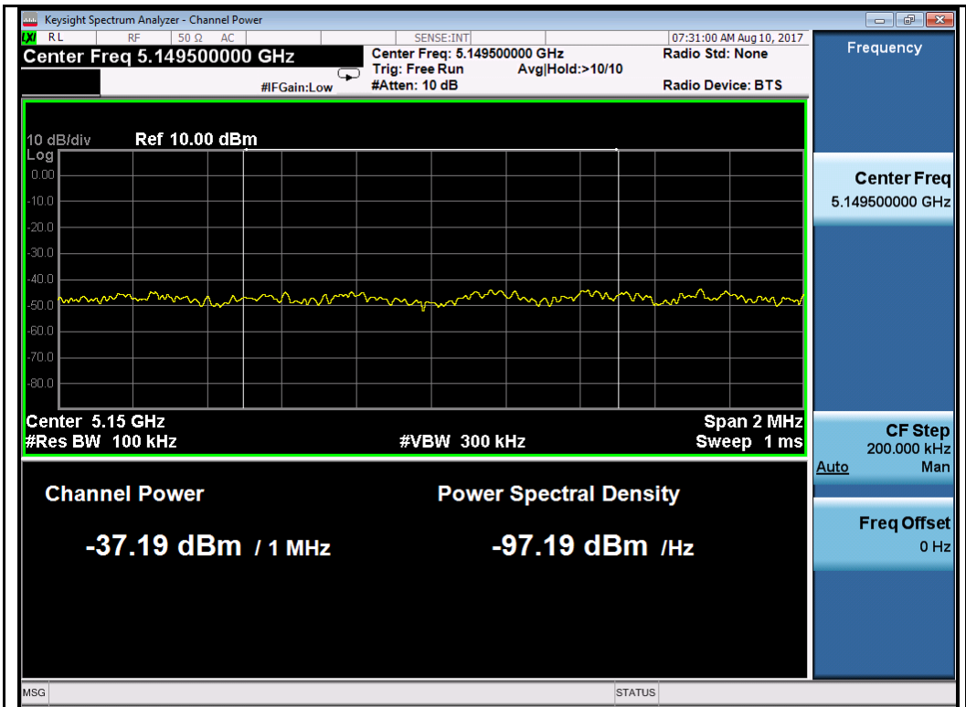
802.11n-HT40-5190MHz
