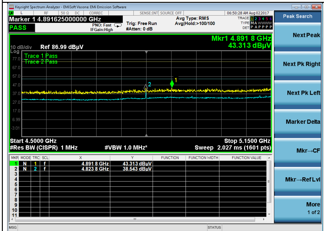
802.11ac-VHT80 5210MHz
