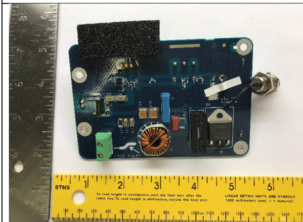
Bias-T Top View
