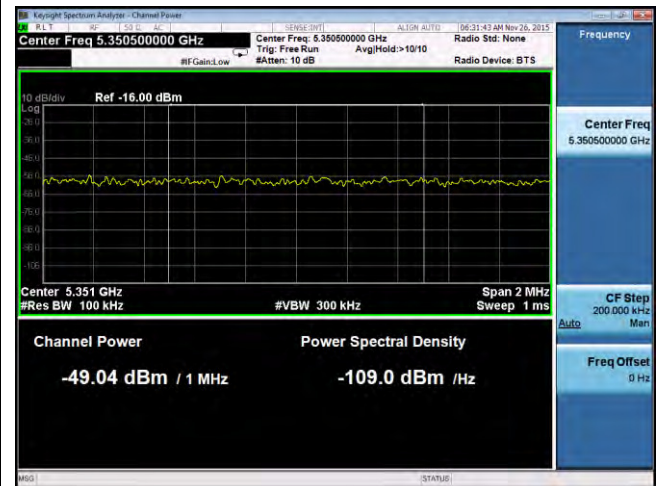
Band Edge -802.11n-20M-5320M-chain4
