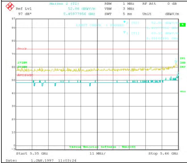
802.11n-HT40 5510M(5350-5460MHz)
