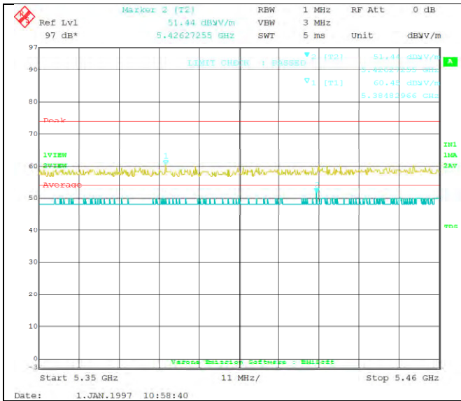
802.11a 5500M(5350-5460MHz)
