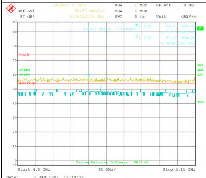
802.11n-HT20 5180M
