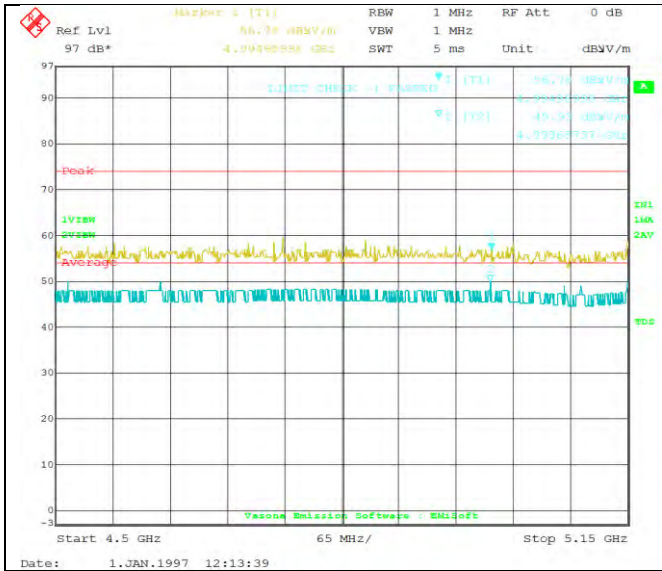
802.11a 5180M
