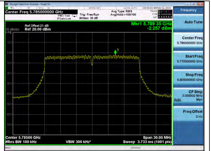
PSD-802.11n-20M-5785M-chain4
