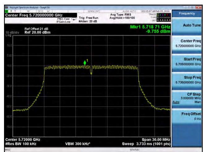
PSD-802.11n-20M-CROSS-5720M-chain4
