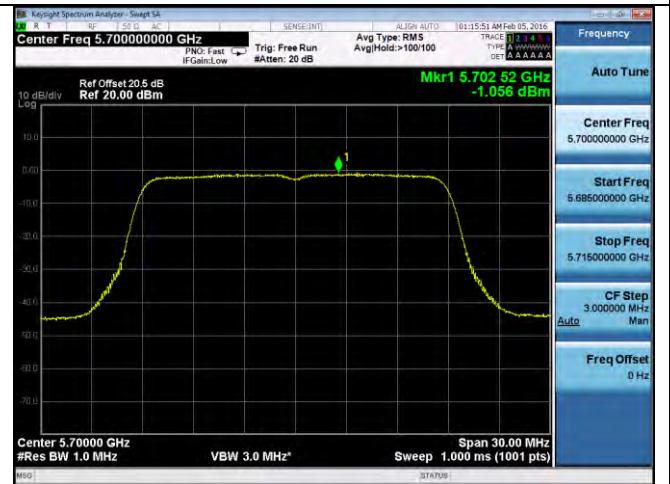
PSD-802.11n-20M-5700M-chain2
