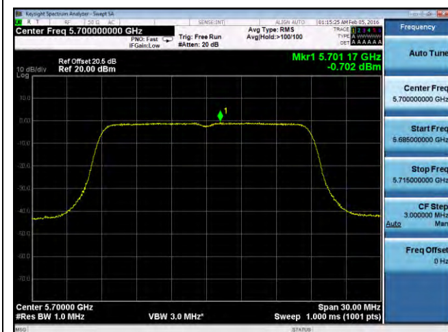
PSD-802.11n-20M-5700M-chain3
