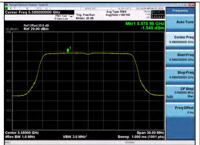
PSD-802.11n-20M-5580M-chain4
