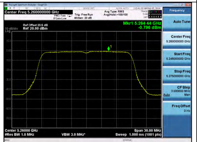
PSD-802.11n-20M-5260M-chain4
