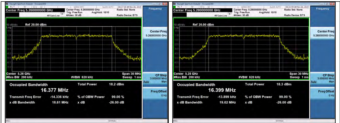
26dB BW -802.11a 5260MHz
