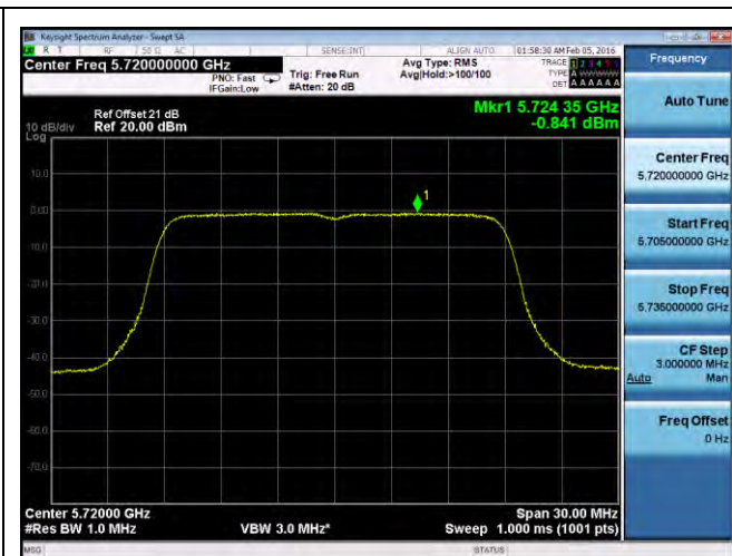
PSD-802.11n-20M-CROSS-5720M-chain4
