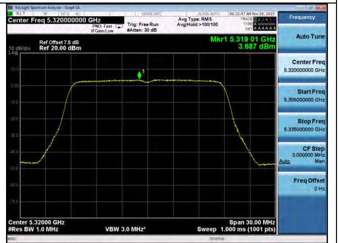
PSD-802.11n-20M-5320M-chain2
