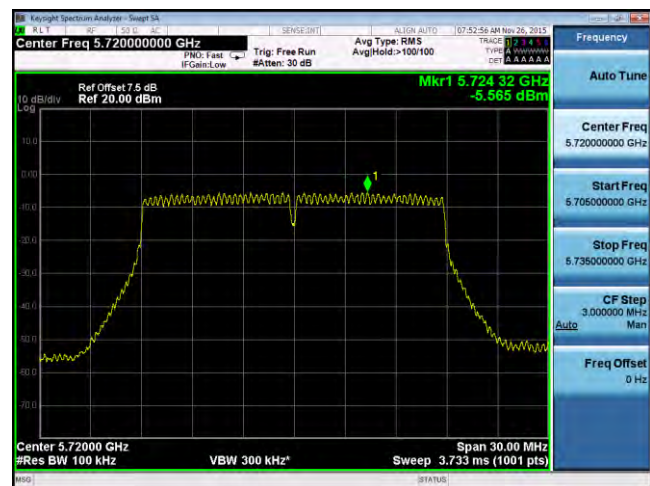
PSD-802.11n-20M-CROSS-5720M-chain4
