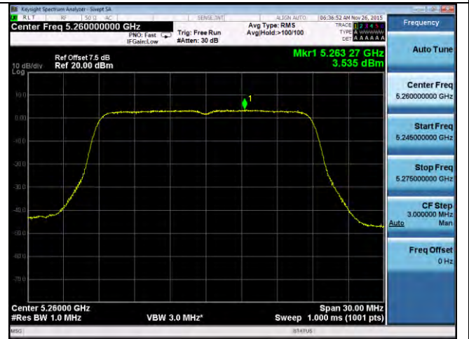
PSD-802.11n-20M-5260M-chain4
