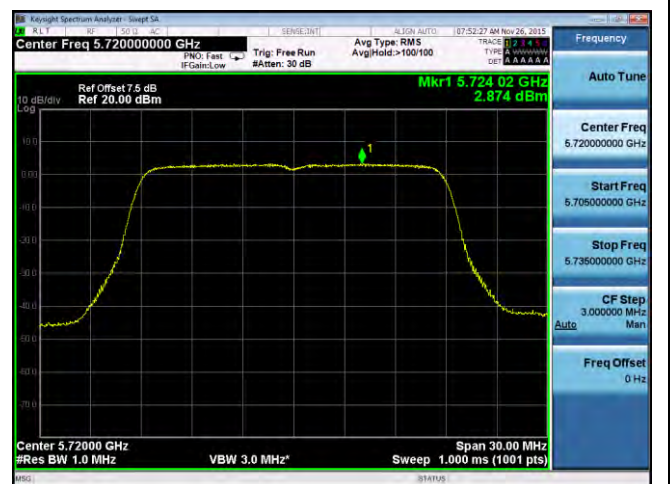
PSD-802.11n-20M-CROSS-5720M-chain4
