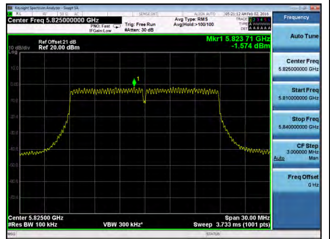
PSD-802.11n-20M-5825M-chain4
