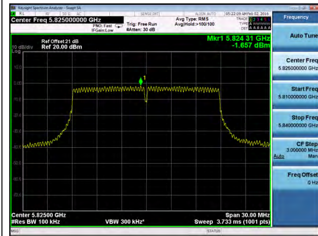
PSD-802.11n-20M-5825M-chain3
