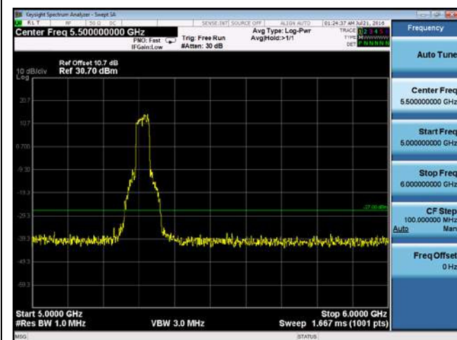
CUE-802.11n-40-5270M-chain3(5GHz-6GHz)
