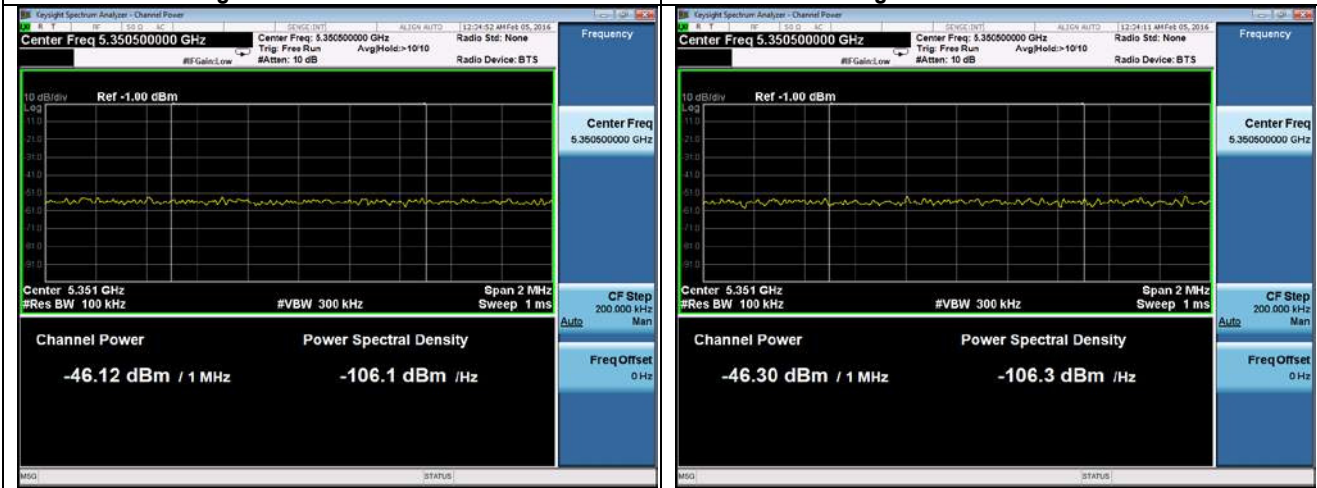
Band Edge -802.11n-20M-5320M-chain3
