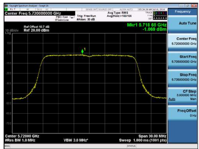
PSD-802.11n-20M-CROSS-5720M-chain4
