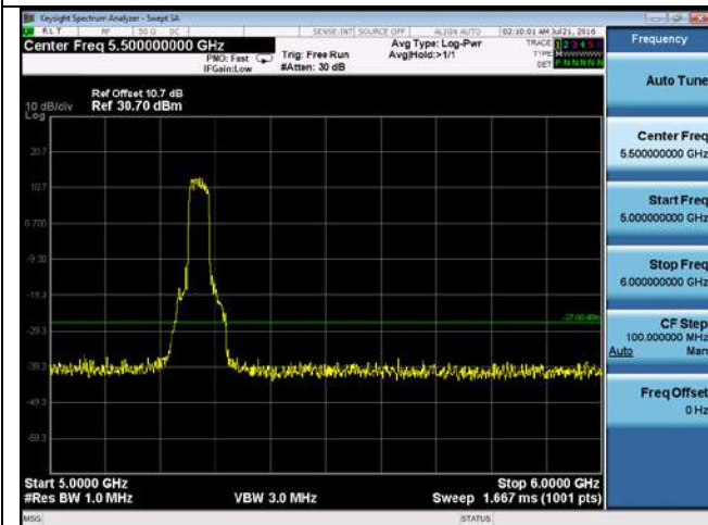
CUE-802.11n-40-5270M-chain4(5GHz-6GHz)
