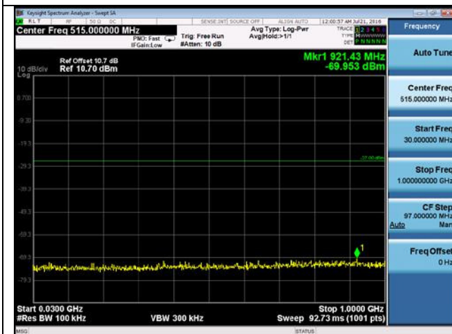
CUE-802.11ac-80-5210M-chain 1(30MHz-1GHz)
