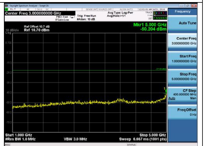
CUE-802.11ac-80-5210M -chain 1(1GHz-5GHz)
