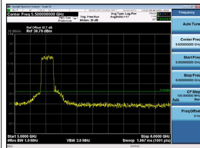
CUE-802.11ac-80-5210M -chain 1(5GHz-6GHz)
