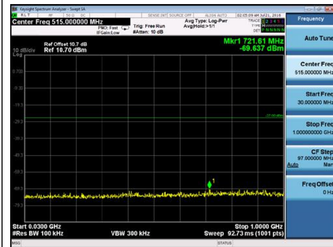
CUE-802.11n-20-5785M -chain4(30MHz-1GHz)
