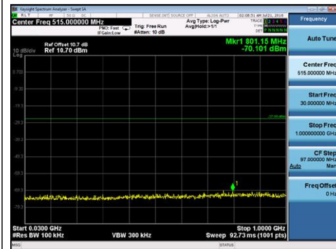
CUE-802.11n-40-5230M -chain4(30MHz-1GHz)
