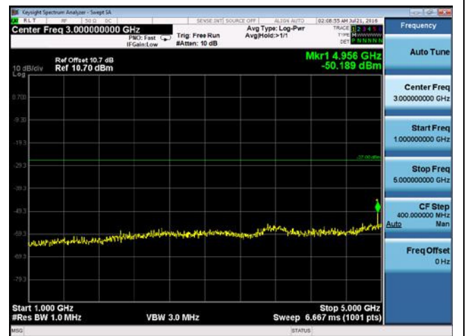
CUE-802.11n-40-5230M -chain4(1GHz-5GHz)
