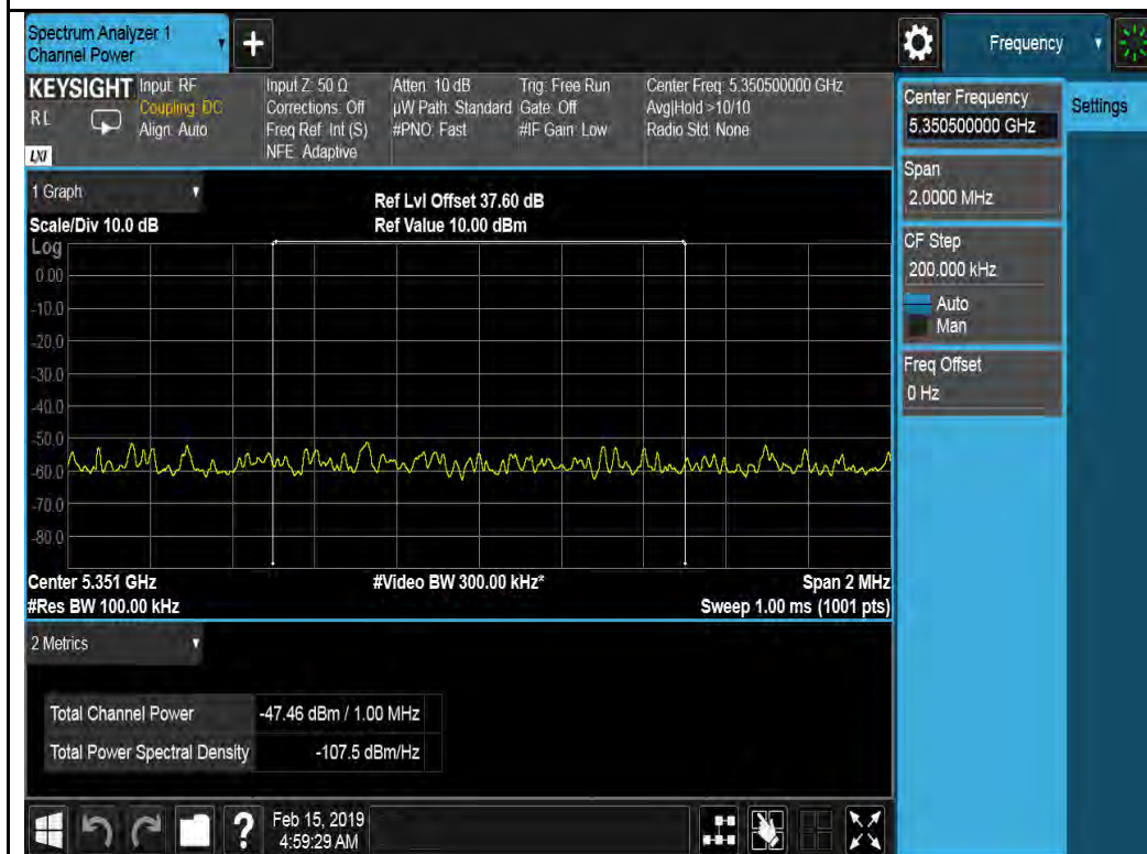
802.11ax-HT40-5310MHz
