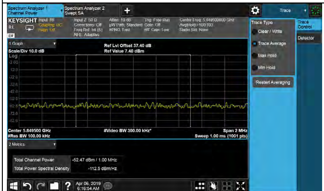
802.11n-5720MHz
