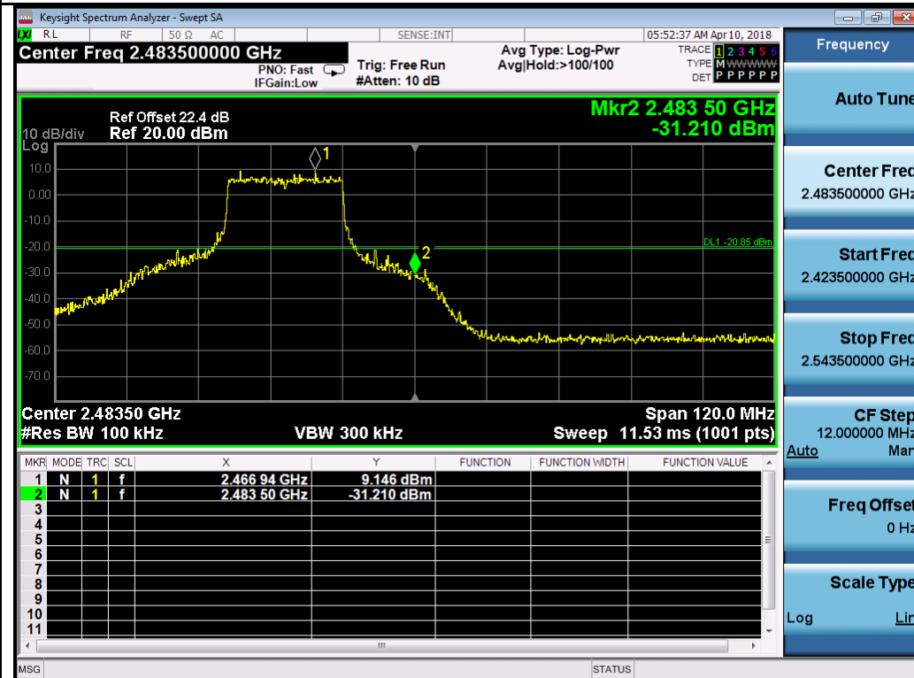
802.11ax20-2462MHz Chain 3
