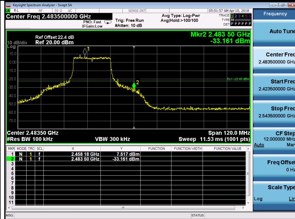
802.11ax20-2462MHz Chain 2
