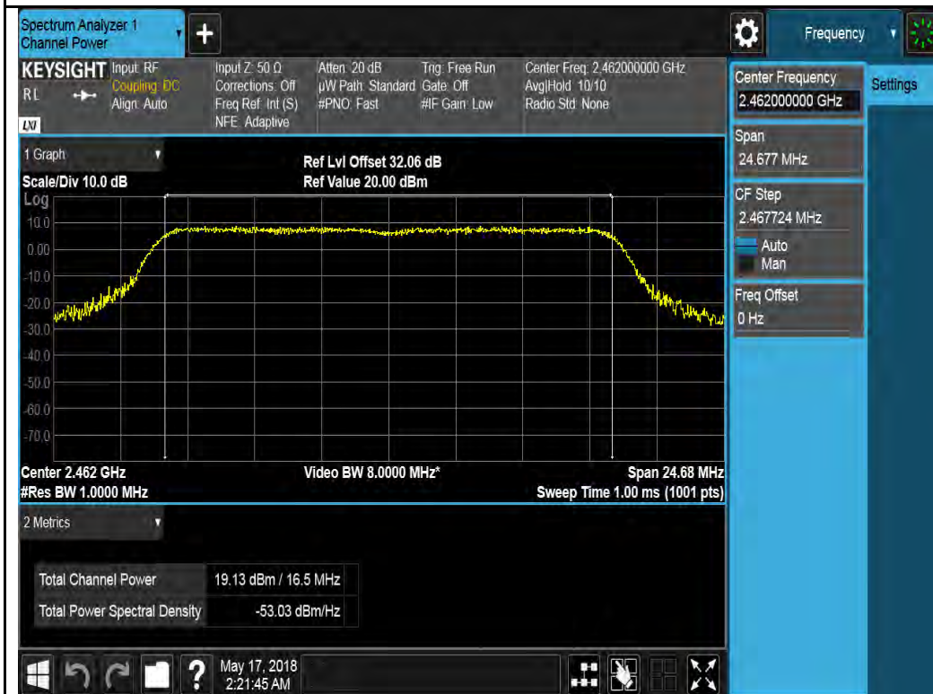
802.11g-2462MHz Chain 3
