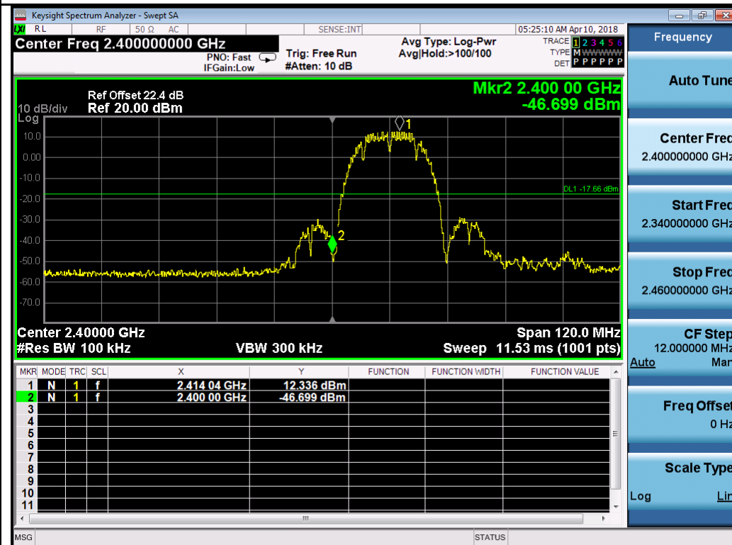
802.11b-2412MHz Chain 3
