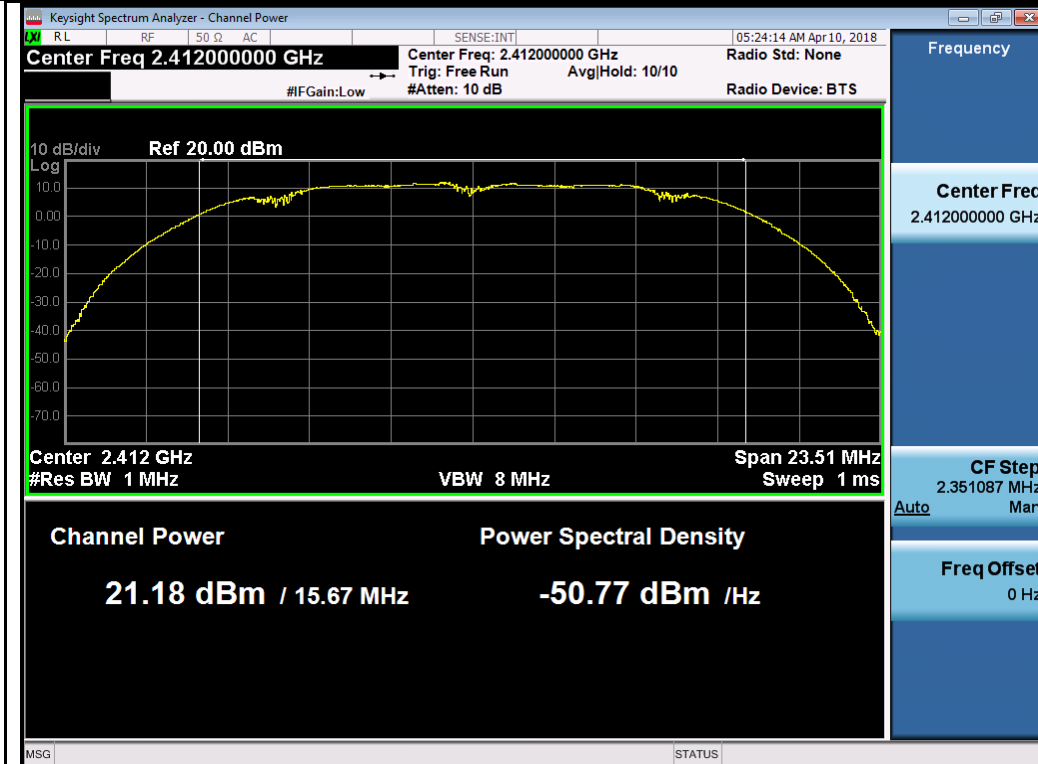
802.11b-2412MHz Chain 2
