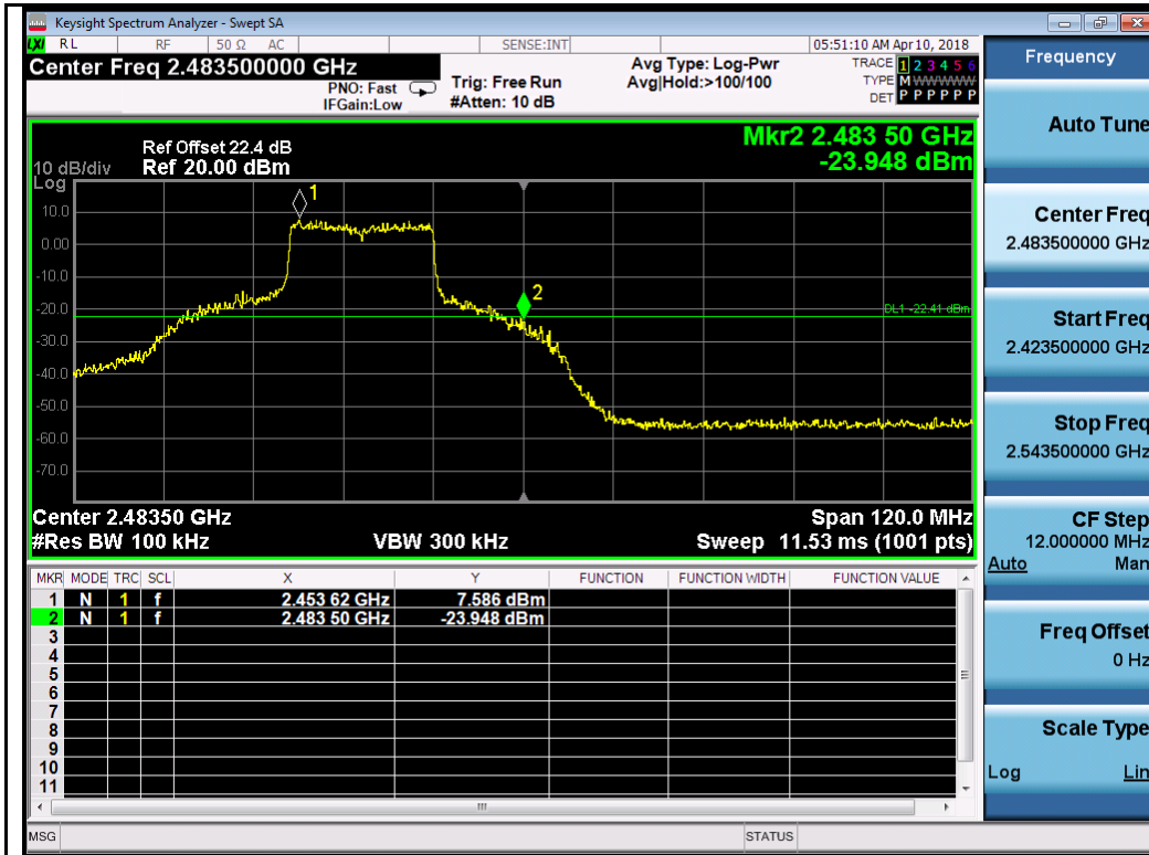
802.11ax20-2462MHz Chain 0
