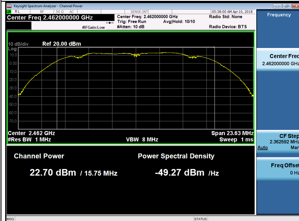
802.11b-2462MHz Chain 3
