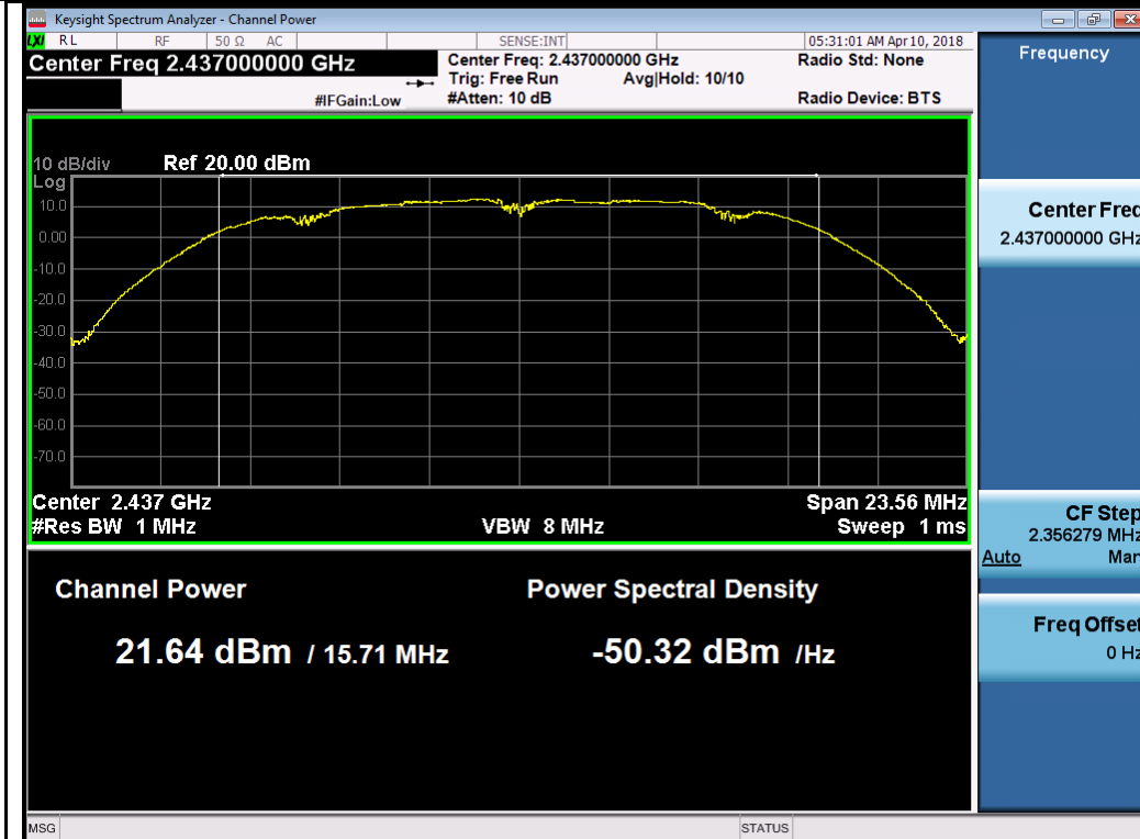
802.11b-2437MHz Chain 0
