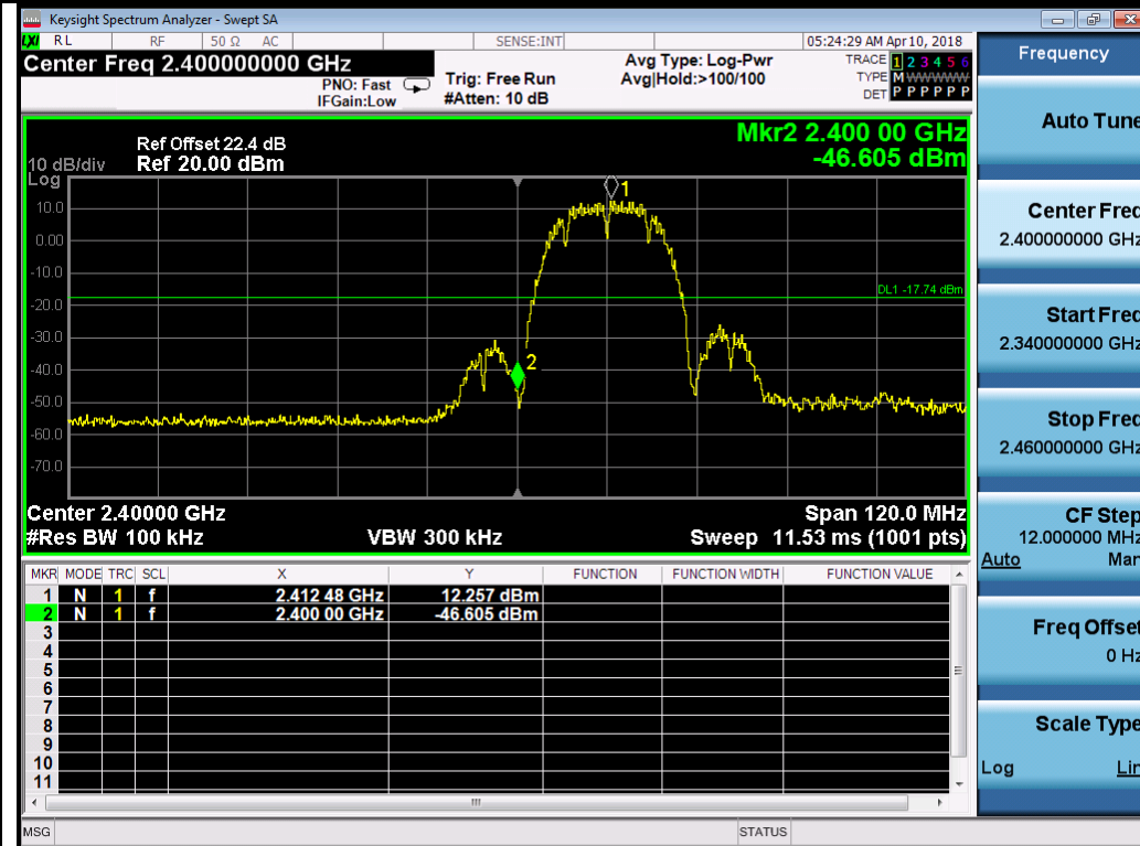
802.11b-2412MHz Chain 2
