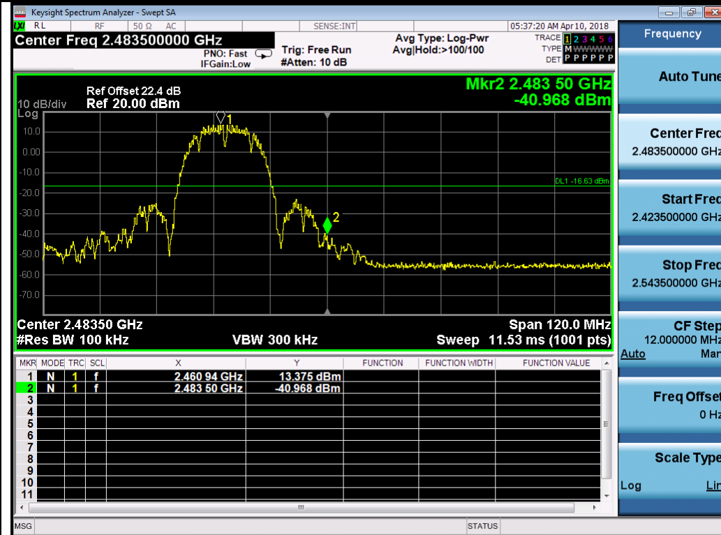
802.11b-2462MHz Chain 2
