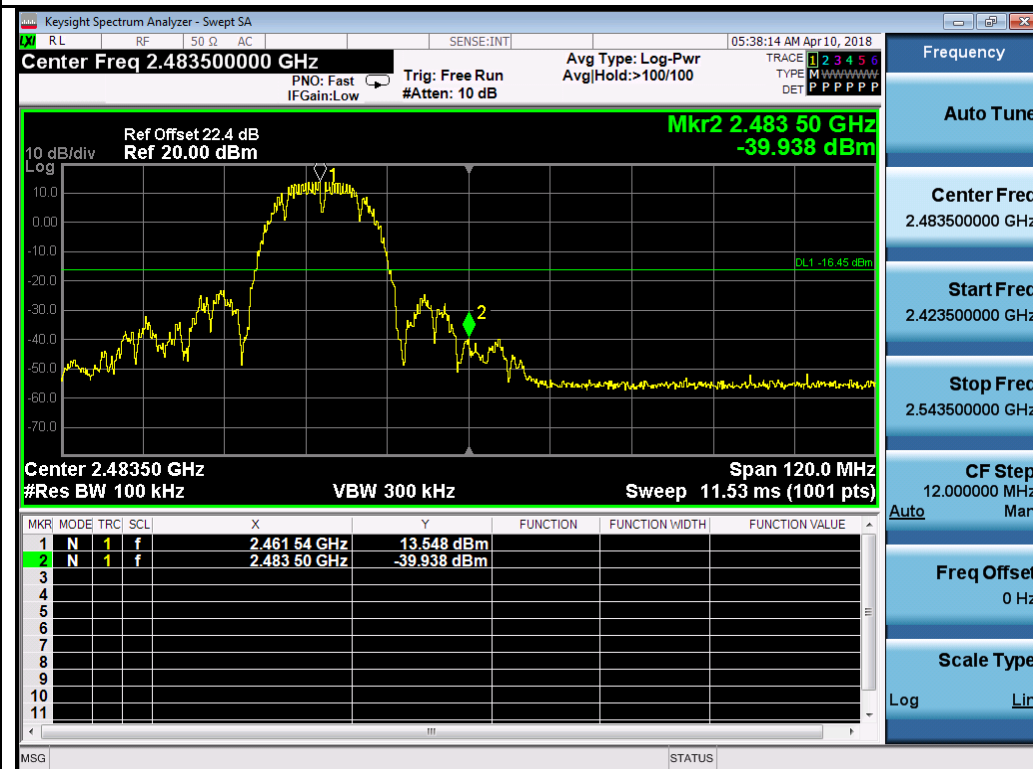
802.11b-2462MHz Chain 3
