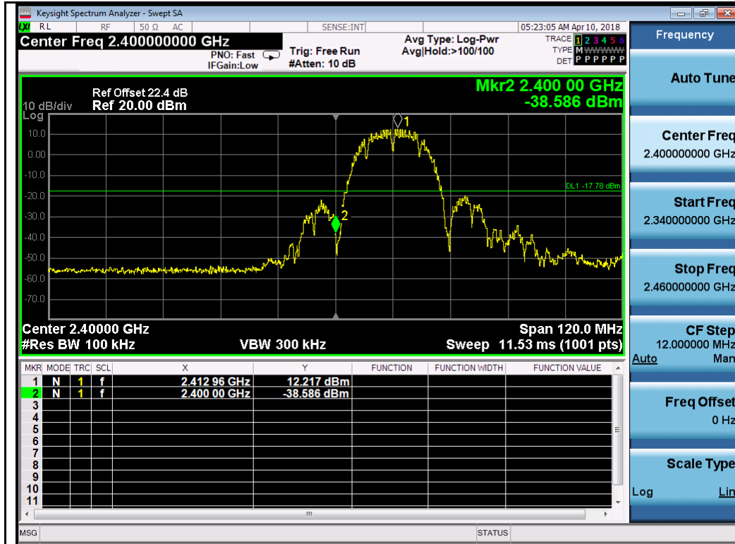
802.11b-2412MHz Chain 0
