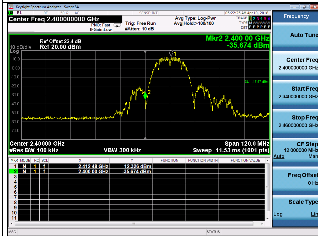
802.11b-2412MHz Chain 1
