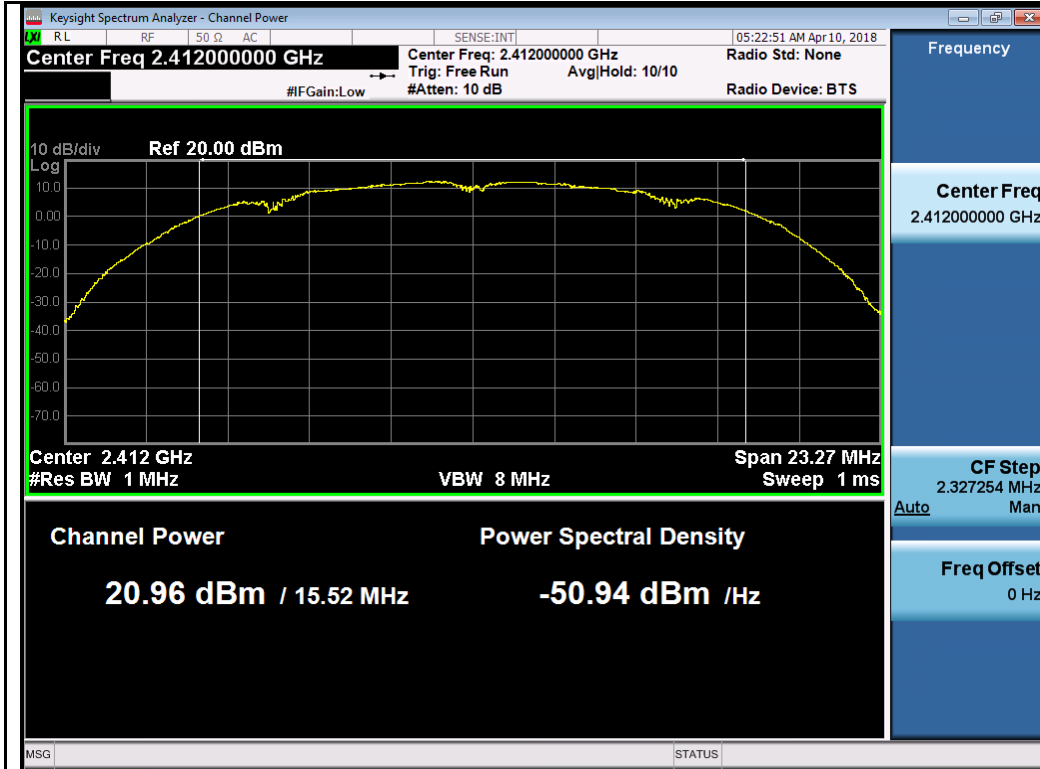
802.11b-2412MHz Chain 0
