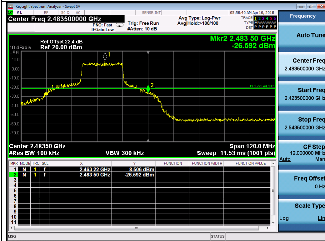
802.11ax20-2462MHz Chain 1
