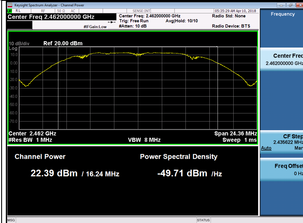
802.11b-2462MHz Chain 0
