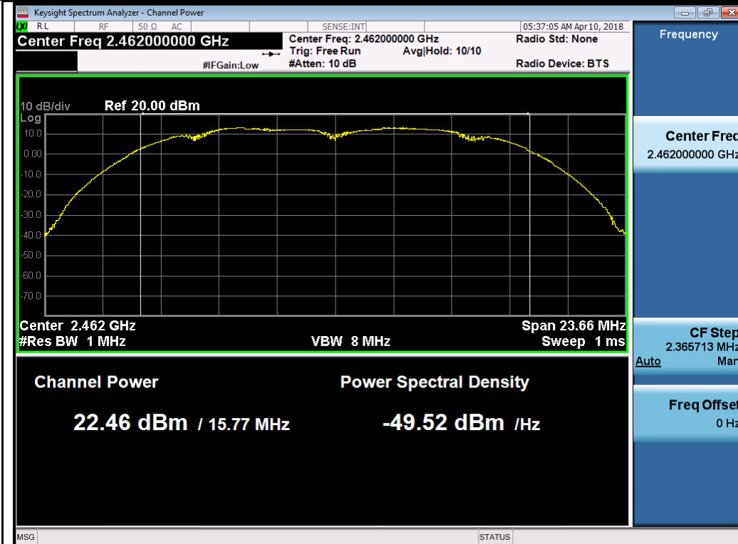
802.11b-2462MHz Chain 2
