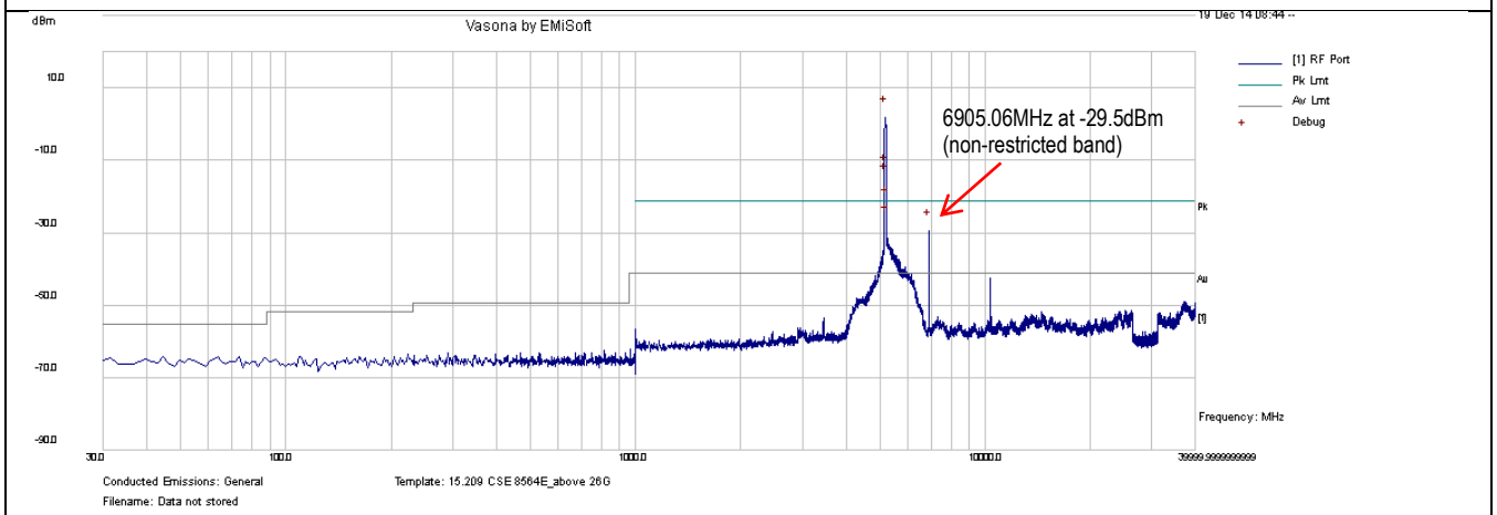
CSE-802.11a 5180MHz-chain1
