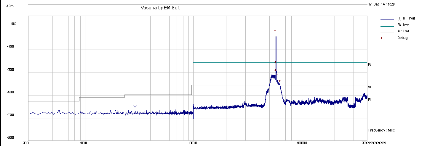
CSE-802.11a 5745MHz-chain1
