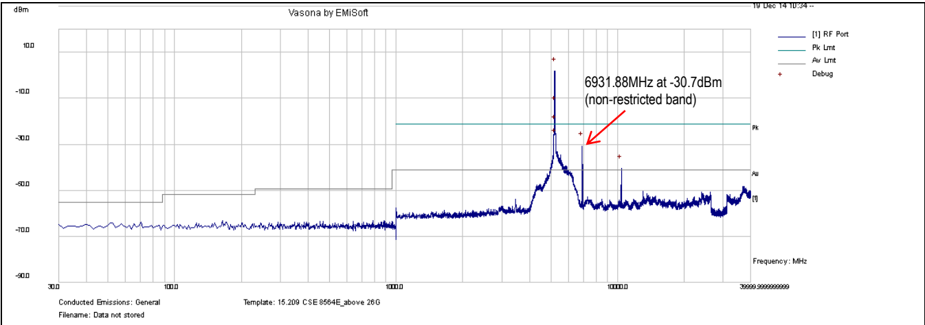
CSE-802.11n-20M 5200MHz-chain1
