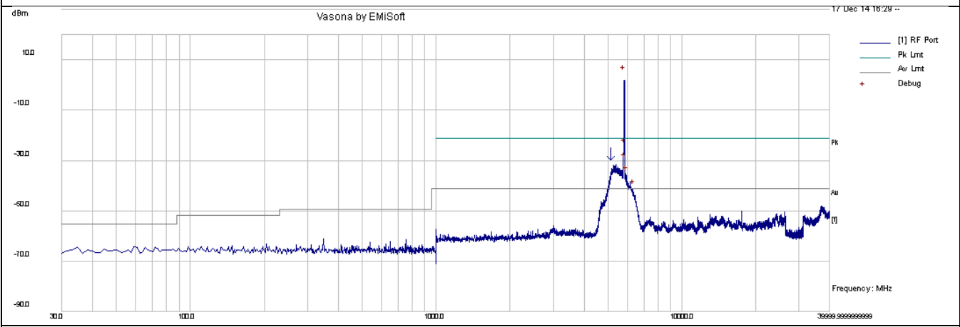
CSE-802.11a 5825MHz-chain1
