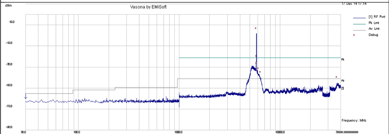
CSE-802.11n-20M 5825MHz-chain1
