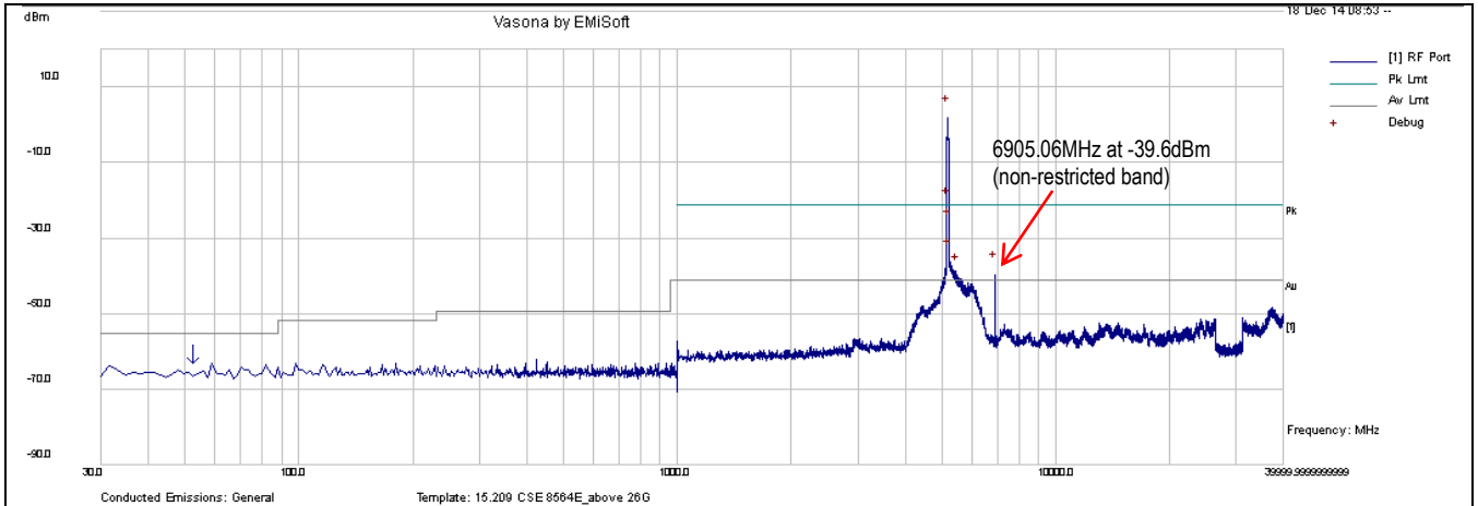
CSE-802.11a 5180MHz-chain0
