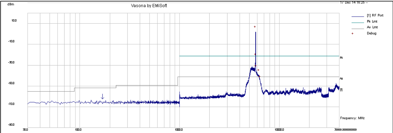
CSE-802.11a 5785MHz-chain1
