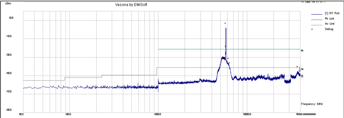
CSE-802.11n-20M 5785MHz-chain1
