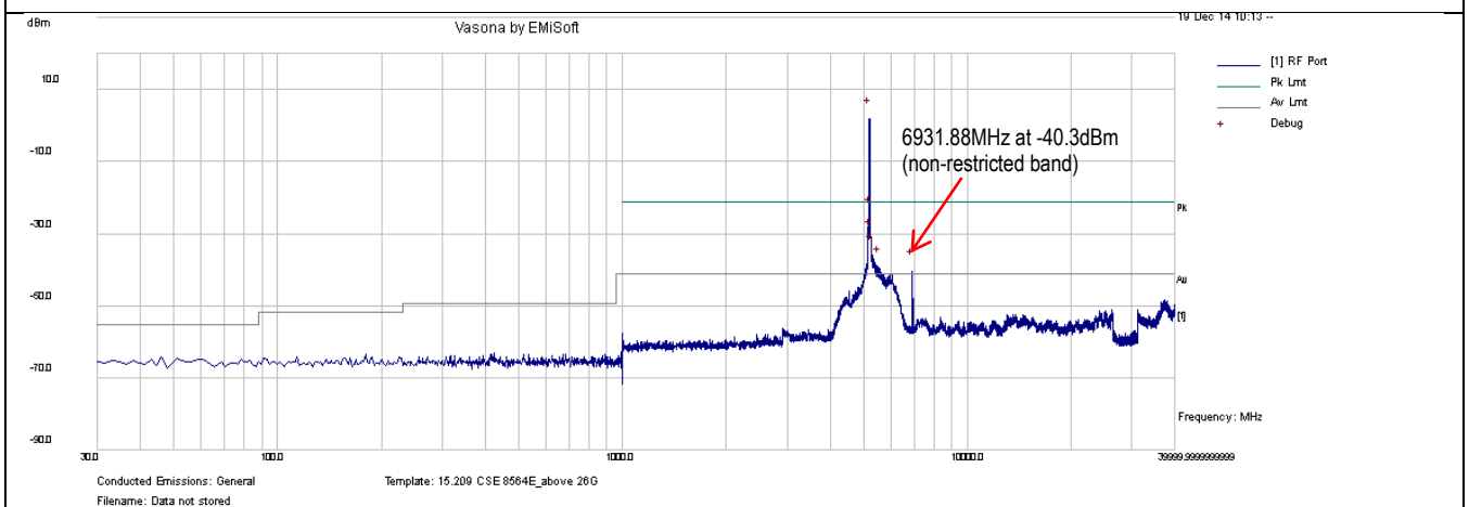
CSE-802.11a 5200MHz-chain0
