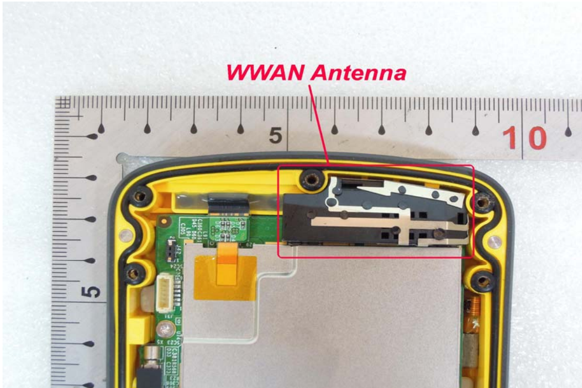
WWAN Antenna - 1
