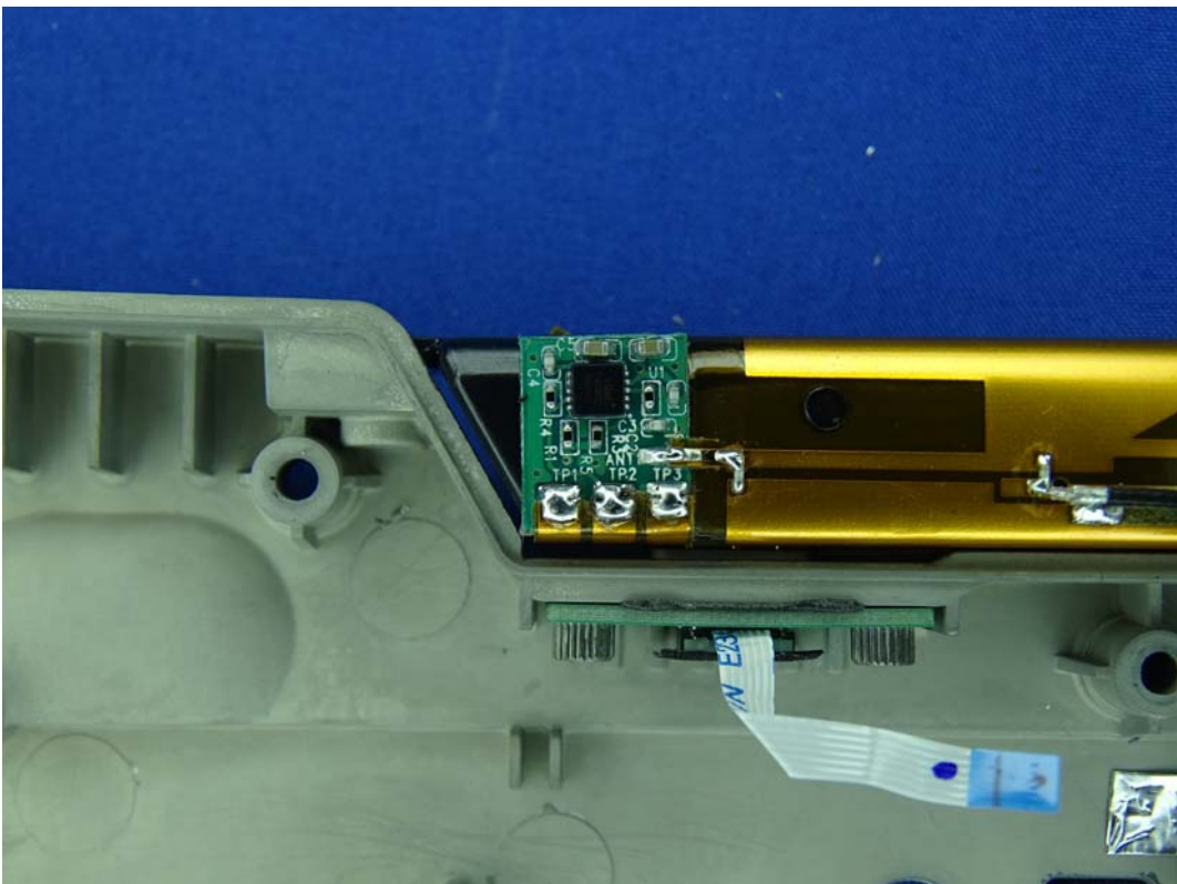
(78) EUT Photo
