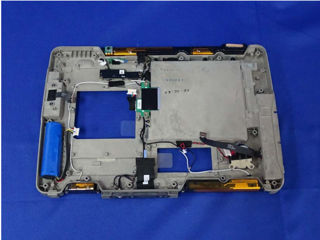
(71) EUT Photo
