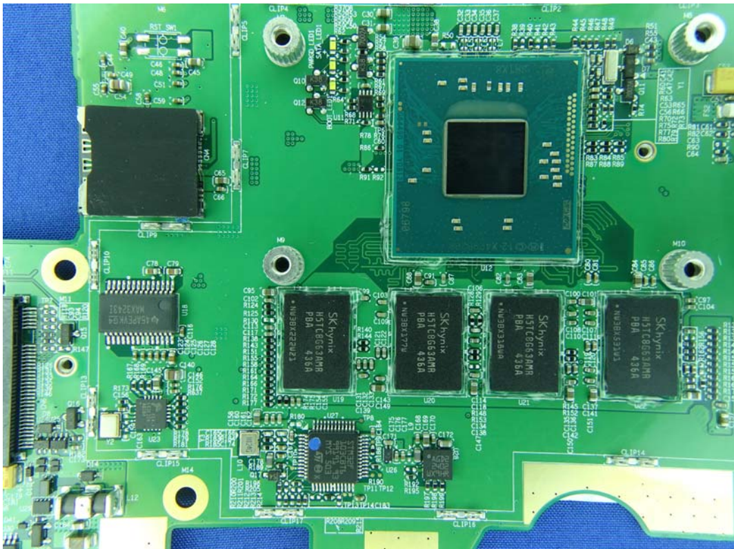
(69) EUT Photo
