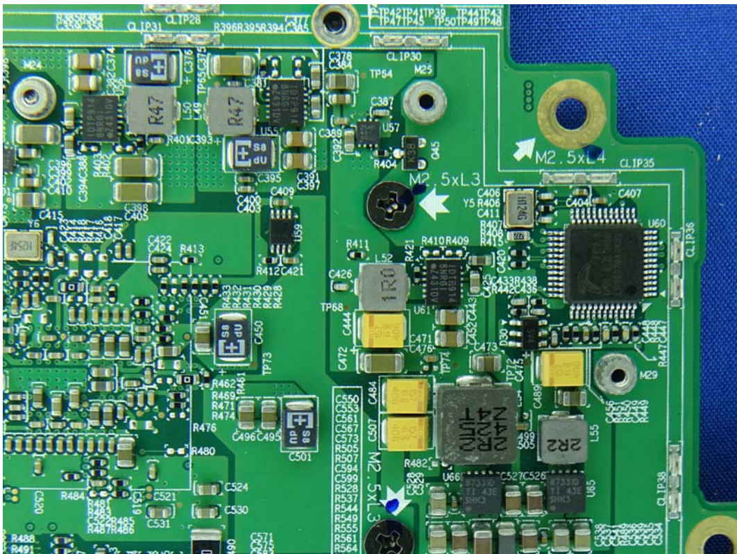
(58) EUT Photo
