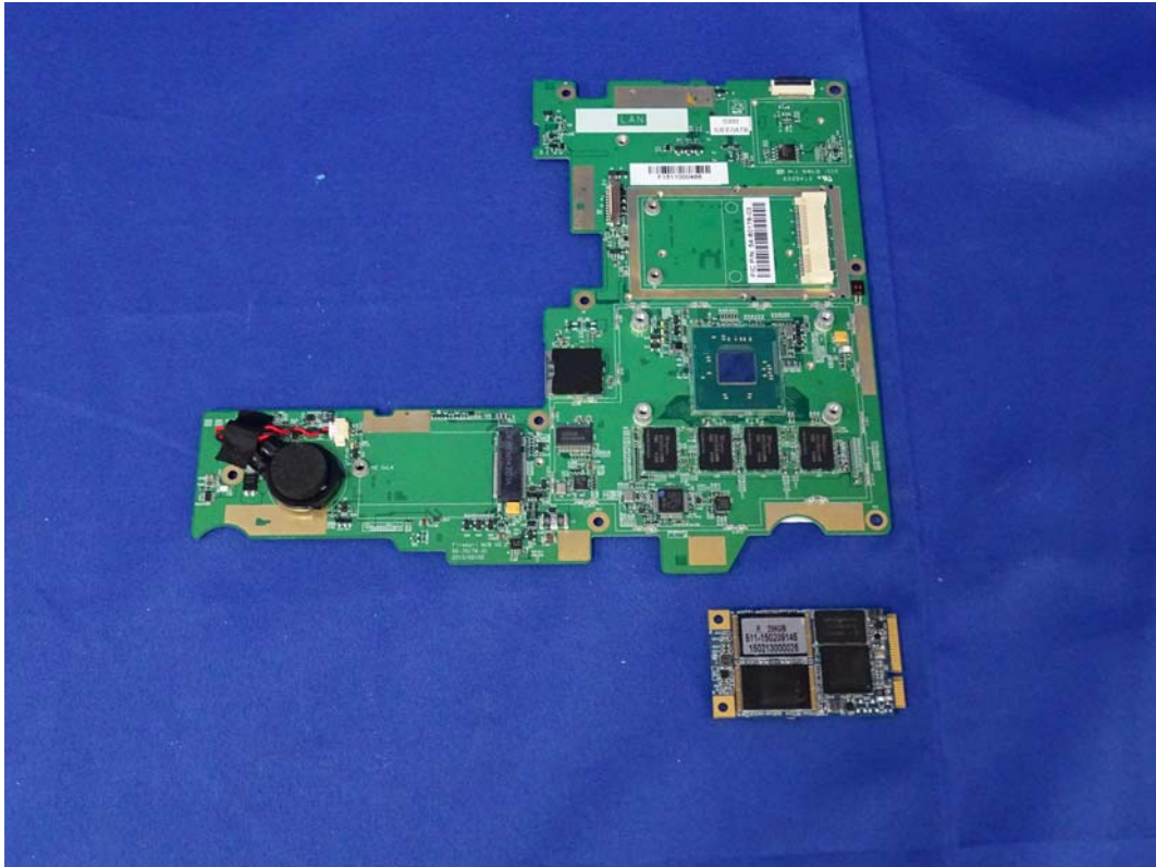
(63) EUT Photo
