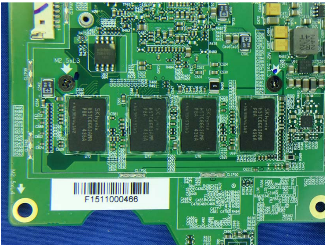
(56) EUT Photo
