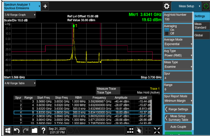
1RB#0 CH 643200 (3648 MHz)
