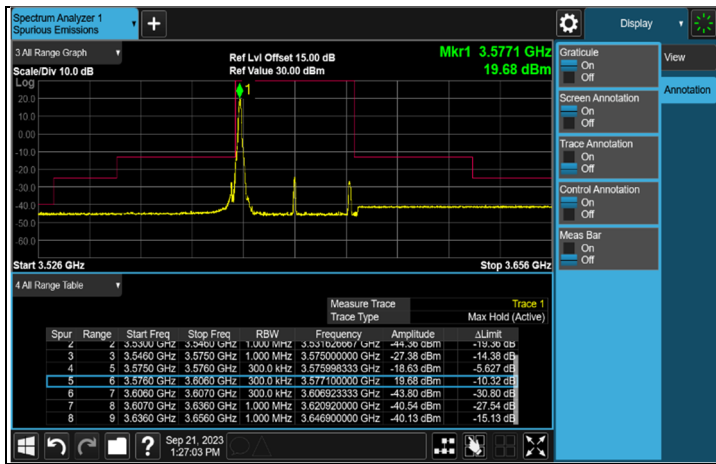
1RB#0 CH 639400 (3591 MHz)
