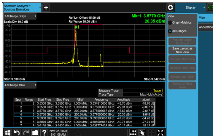
1RB#0 CH 639068 (3586.02 MHz)
