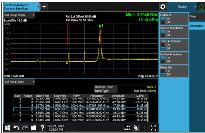
1RB#MAX CH 639400 (3591 MHz)
