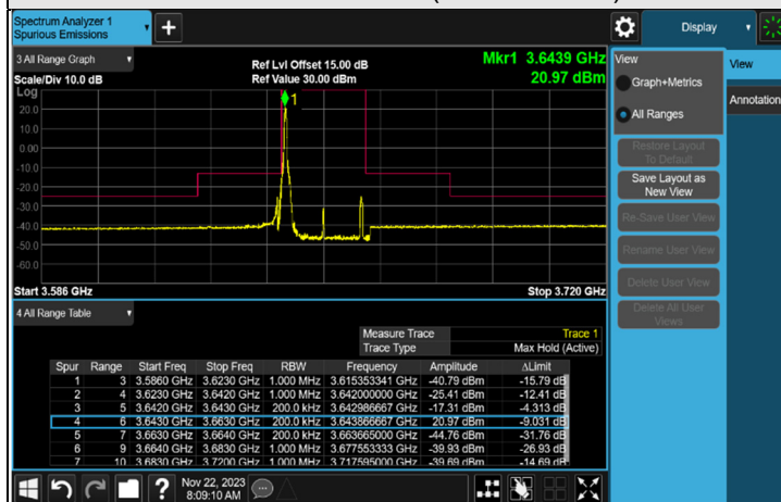
1RB#0 CH 643532 (3652.98 MHz)
