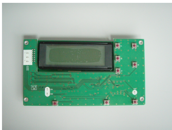
(PCB)
